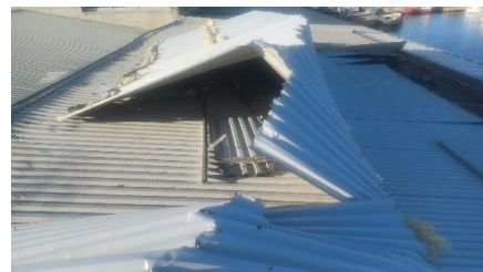
Trams de coberta en procés d'arrencament durant la ventada.
