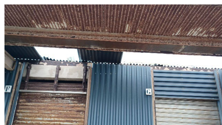
Trams de coberta amb elements despresos i fixacions i elements estructurals descoberts amb un elevat estat de corrosió
