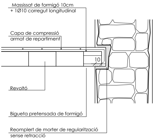
DETALL TROBADA BIGUETA FORJAT-MUR
