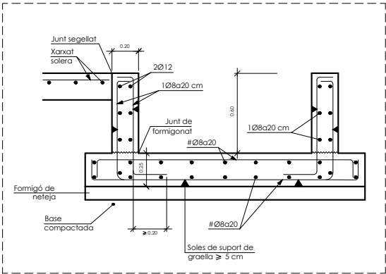
DETALL FOSSAT ASCENSOR
