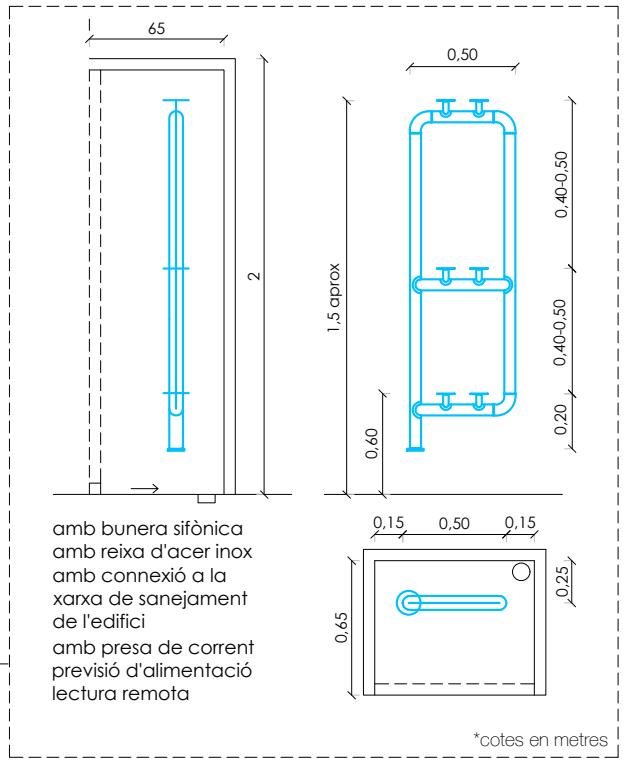
DETALL ARMARI COMPTADORS 3 FILERES 5 SERVEIS
