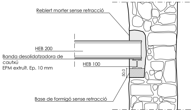
DETALL TROBADA BIGA METÀLICA-MUR FAÇANA
