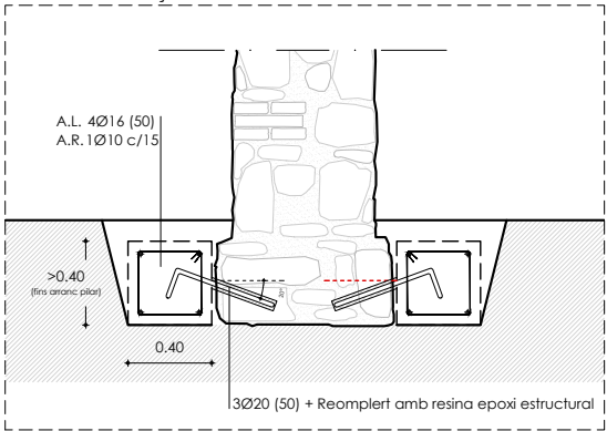
DETALL RECALÇAT PILAR MUR
