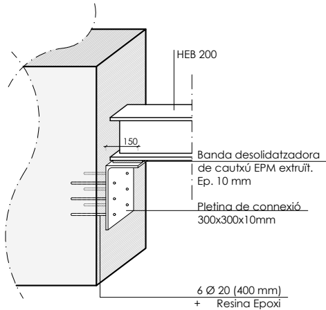
DETALL TROBADA BIGA-PILAR CENTRAL
