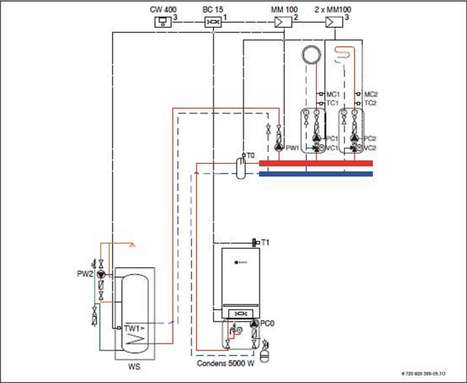
ESQUEMA DE PRINCIPI PER A DOS CIRCUITS DE CALEFACCIÓ AMB VÀLVULA BARREJADORA, UN CIRCUIT PER ACS, COMPENSADOR HIDRAÚLIC I CONTROL PER SONTA EXTERIOR
