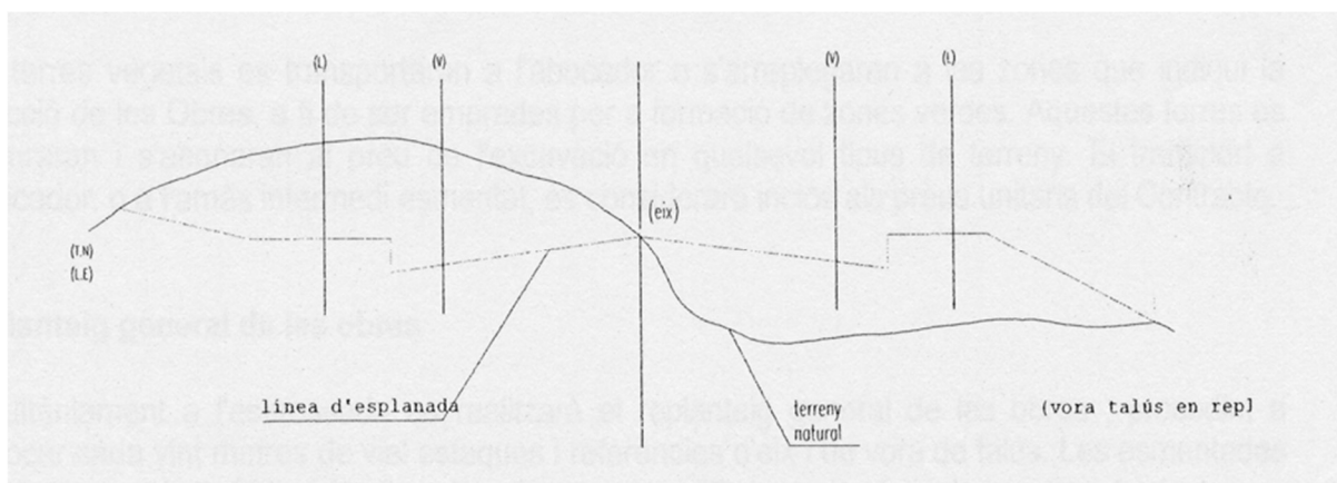
(L) Línia límit d'espai públic – espai parcel·lat (V) Línia de vorada (TN) Terreny natural (LE) Línia d'esbrossada Figura -2-
