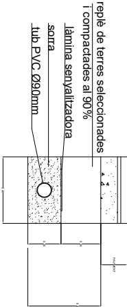
DETALL RASA ENLLUMENAT PÚBLIC
