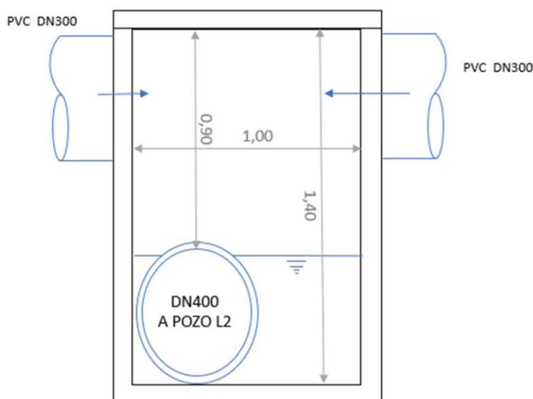
CORTE LONGITUDINAL
