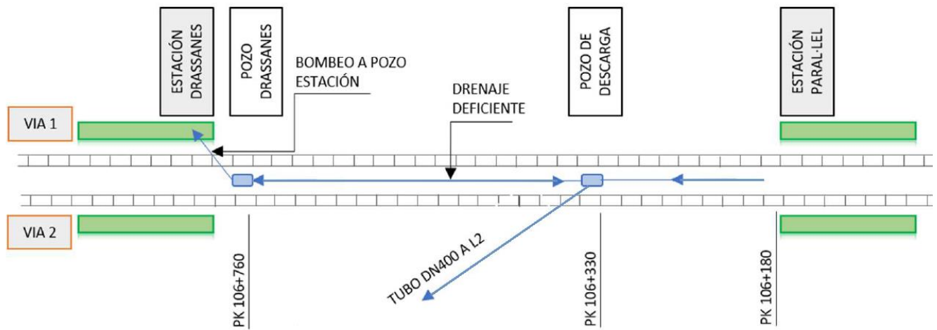
Esquema de drenatge
