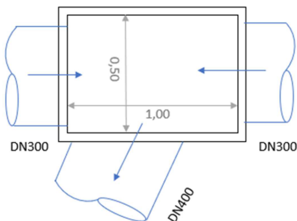
CORTE LONGITUDINAL
