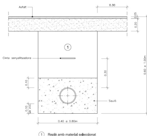
DETALL RASA "TIPUS 1" (Casc urbà o similars) A CALÇADA
