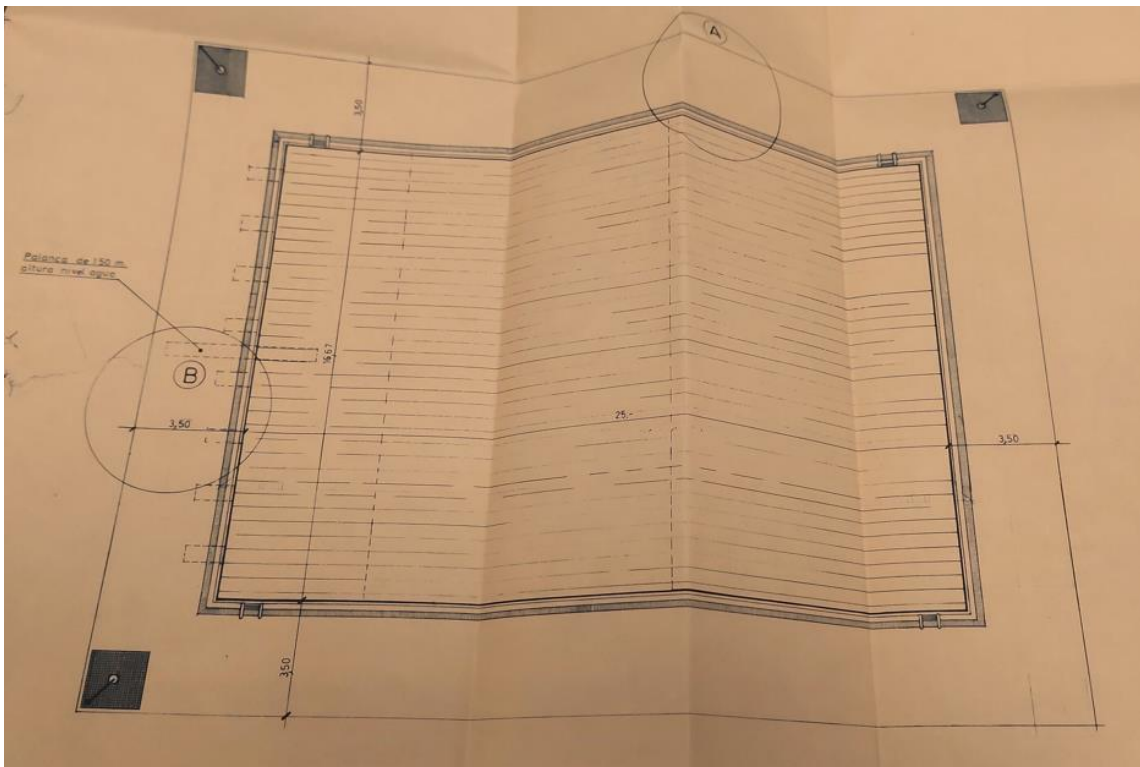
PISCINA D'ADULTS
