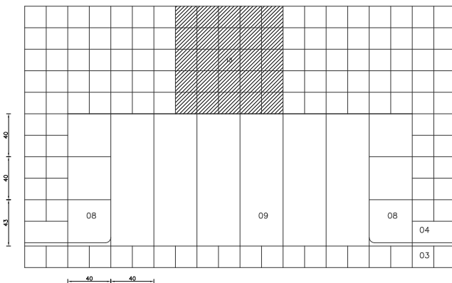
G02 GUAL DE VIANANTS DE GRANIT
