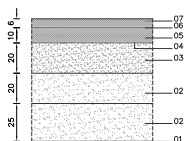
P01 FERM DE PAVIMENT ASFÀLTIC
