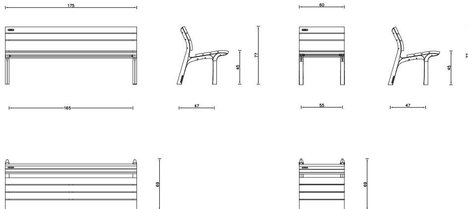
S05 CADIRA NEOROMANTIC 175 D'URBIDERMIS
