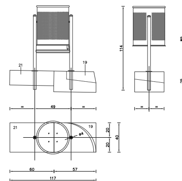
U02 PAPERERA BARCELONA DE 701 DE BENITO
