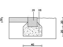
P15 VORADA DE TAUJÓ RECTA DE PECES DE FORMIGÓ DE 20x20cm
