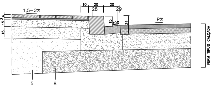
P17 VORADA DE GRANIT
