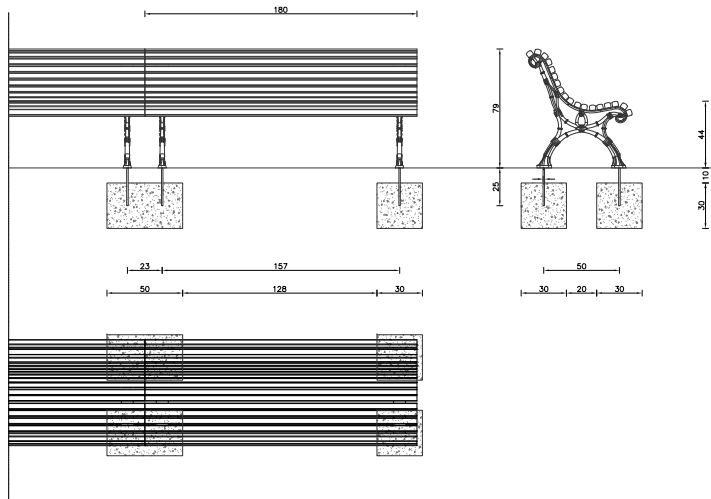
S01 BANÇ BARCINO DE BENITO
