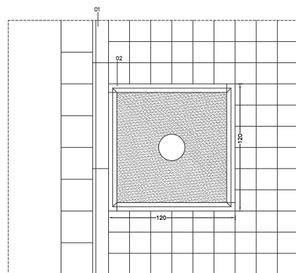
E01 ESCOCELL QUADRAT TIPUS FIOI DE 120X120
