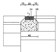
P14 RIGOLA 20cm
