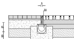
P14 RIGOLA 20cm
