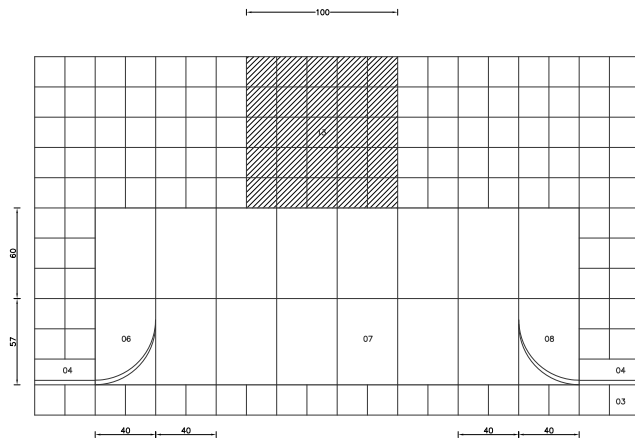
G01 GUAL DE VIANANTS DE FORMIGÓ PREFABRICAT
