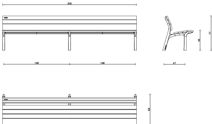
S04 BANÇ NEOROMANTIC 300 D'URBIDERMIS
