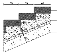
P15 VORADA DE TAUJÓ RECTA DE PECES DE FORMIGÓ DE 20x20cm
