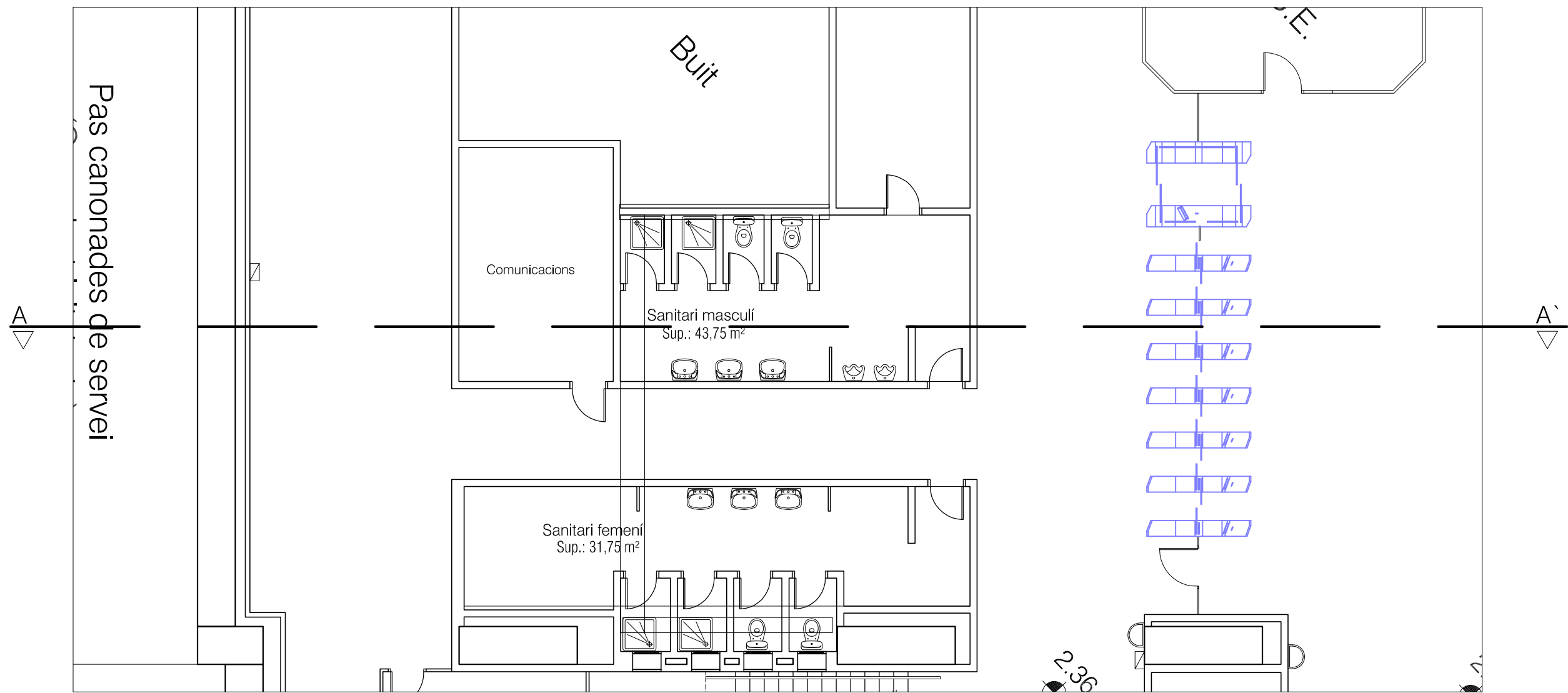
Planta distribució (actual) Escala 1:50
