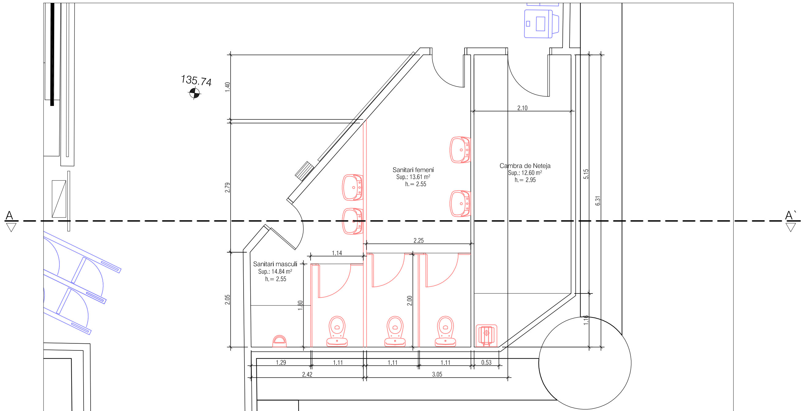
Planta distribució proposta
