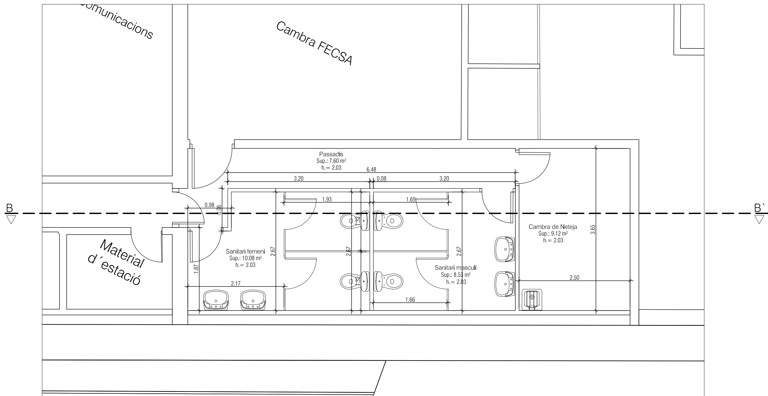
Planta distribució proposta Escala 1:50
