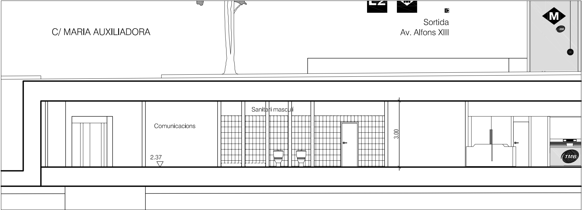
Secció longitudinal A-A' Escala 1:50
