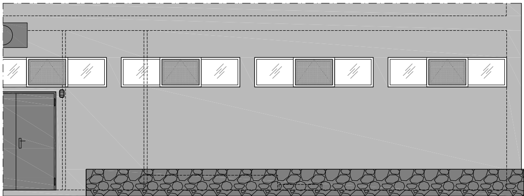
ALÇAT A-A' ESTAT ACTUAL
