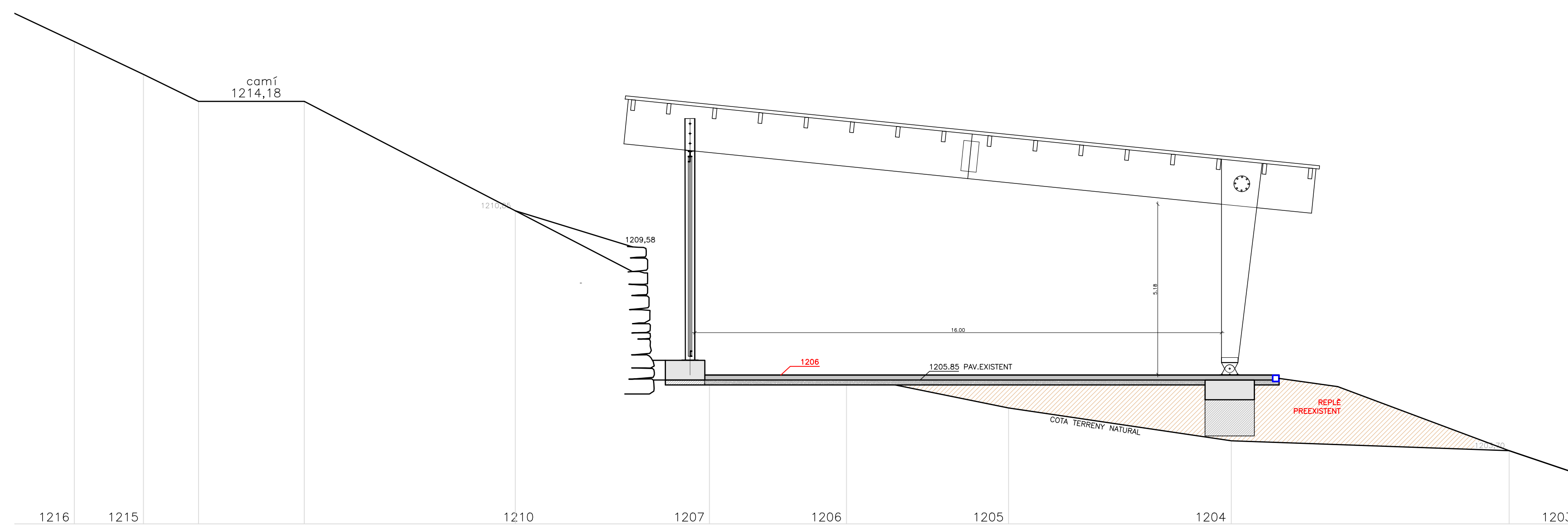
SECCIÓ B
