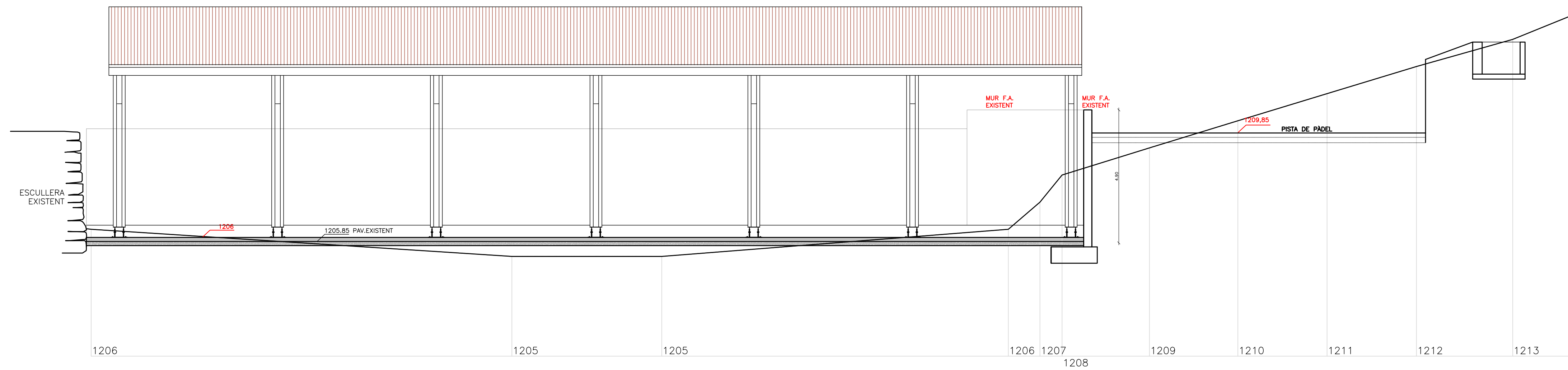
SECCIÓ D
