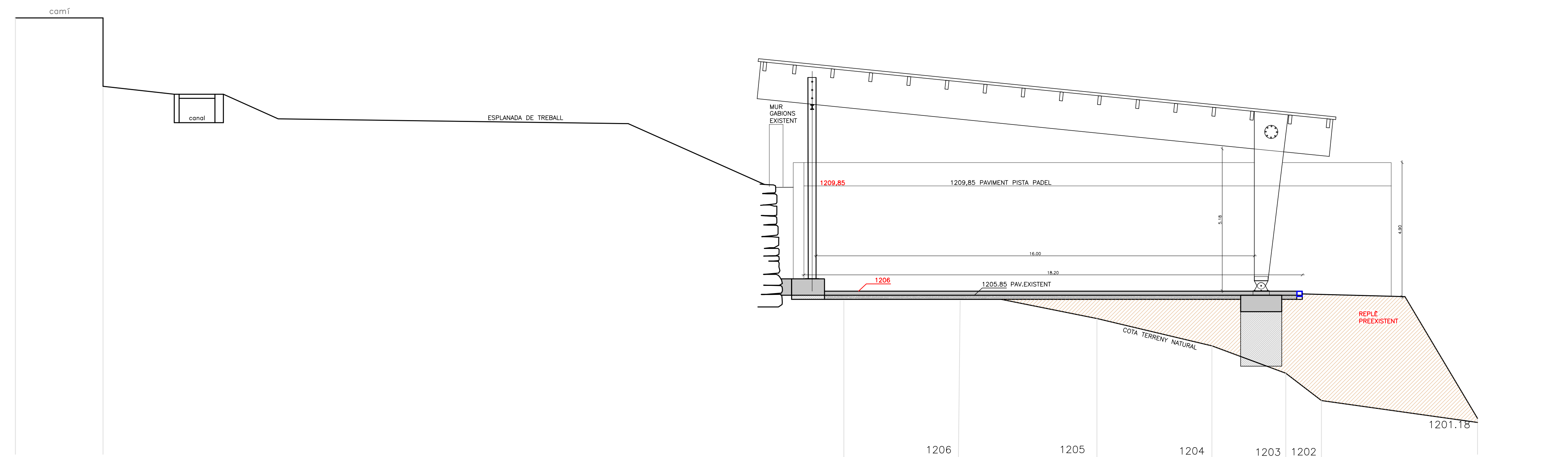
SECCIÓ A
