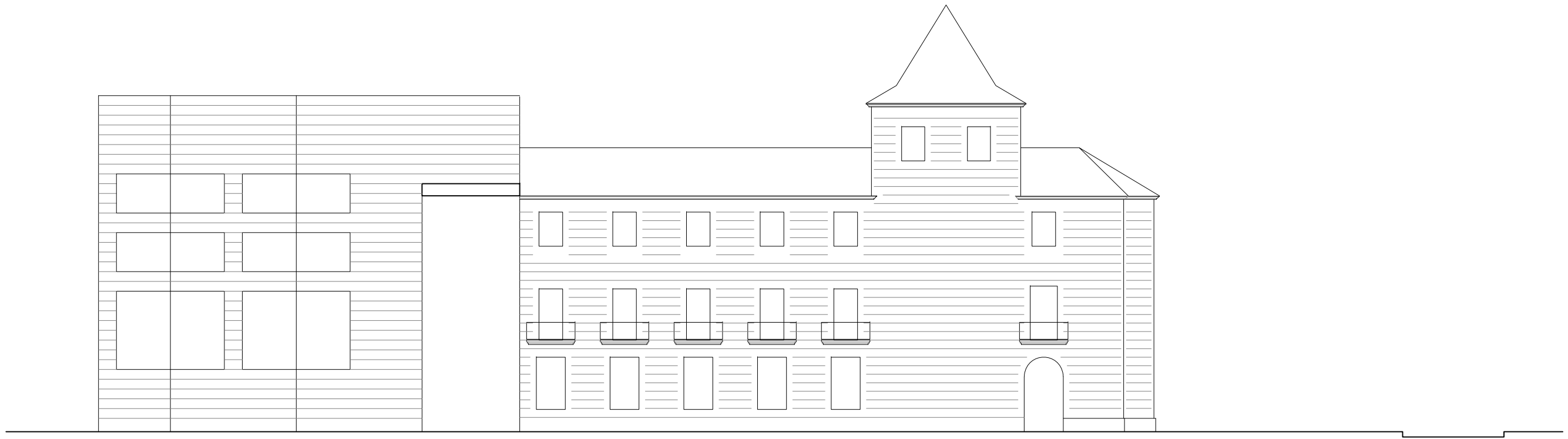
Façana al c. Portal de santa Madrona
