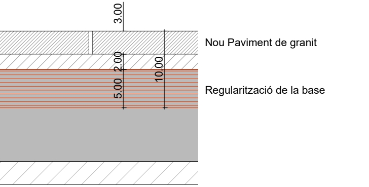
Det 4. Paviment PROPOSTA e 1:5
