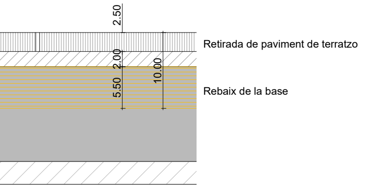
Det 4. Paviment ESTAT ACTUAL e 1:5
