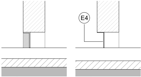
Det 3. Sòcol paraments ESTAT ACTUAL e 1:5
