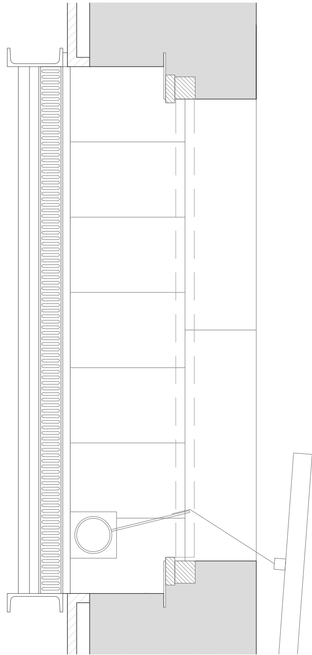
Det 1 ESTAT ACTUAL
