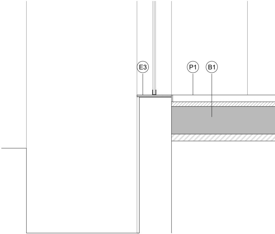
SECCIÓ PROPOSTA
