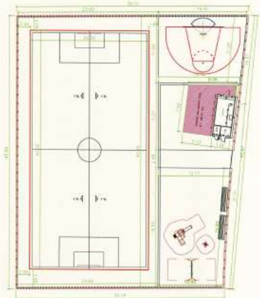
PLANTA SITUACIÓ
