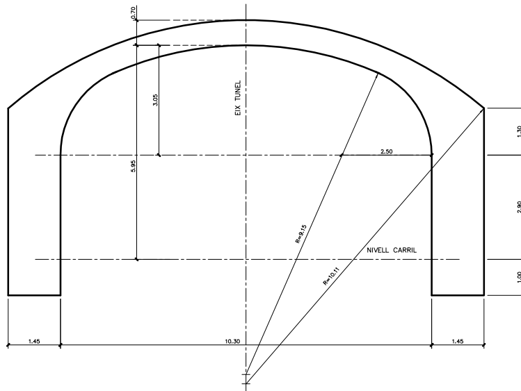
SECCIÓ TUNEL TIPUS 1-S145 ESCALA 1:50
