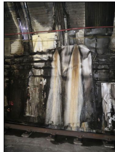
Foto 10: Filtració capcer PK 103+700 via 2
