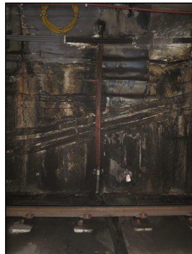
Foto 4: Filtració pantalla PK 103+663 v2.
