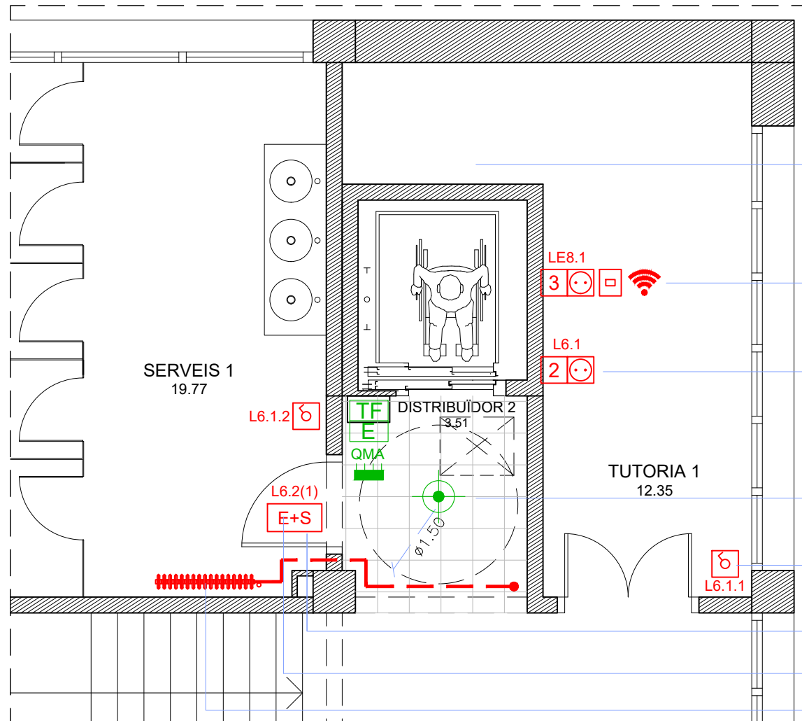
PROPOSTA DISTRIBUCIÓ. PLANTA TERCERA
