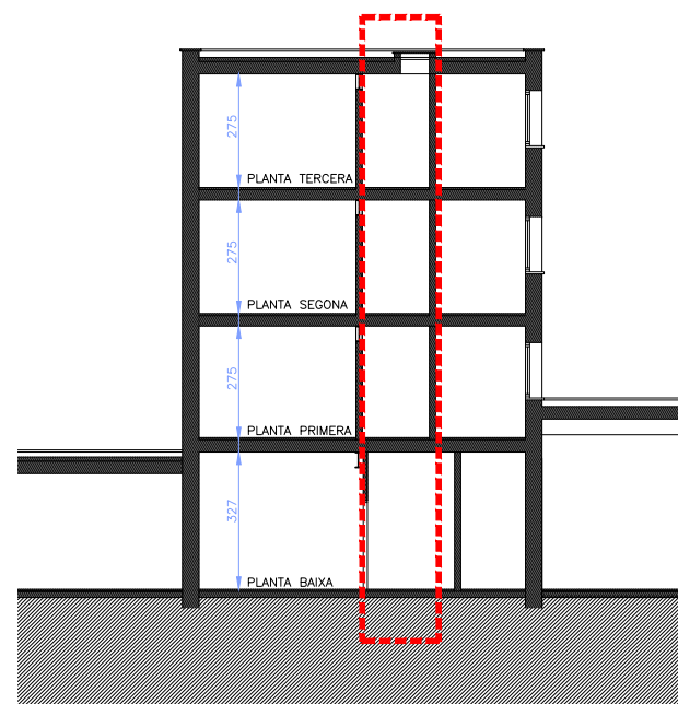
SECCIÓ B-B'
