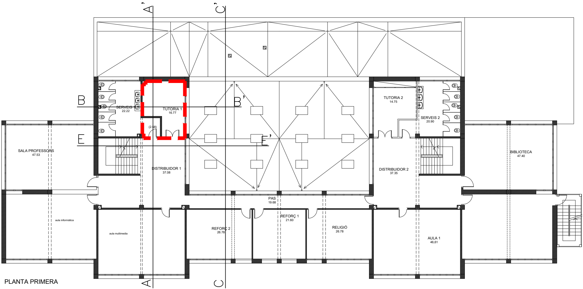
PLANTA BAIXA
