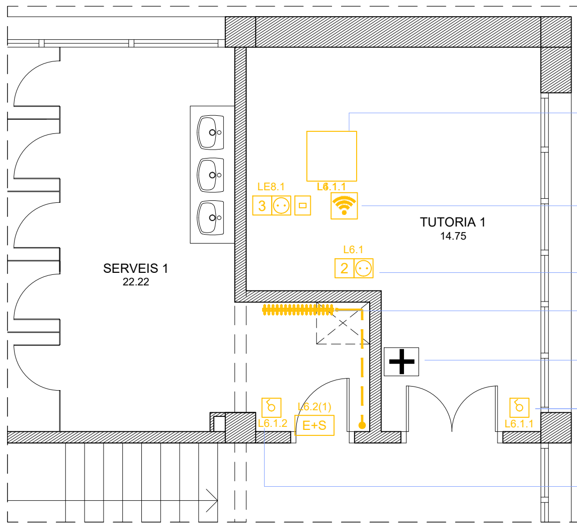
ESTAT ACTUAL. PLANTA TERCERA
