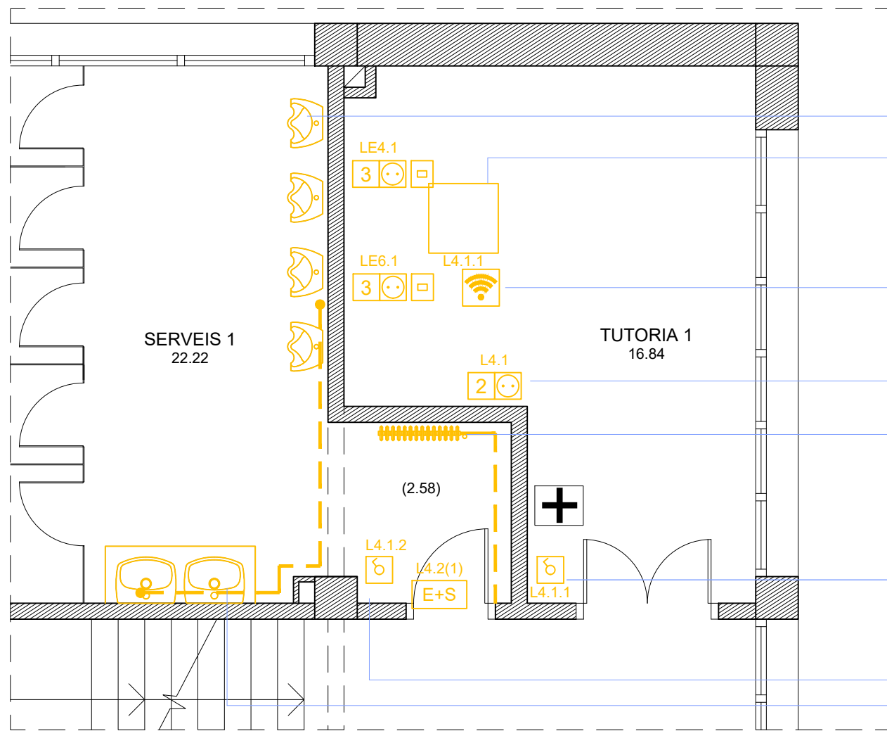
ESTAT ACTUAL. PLANTA SEGONA
