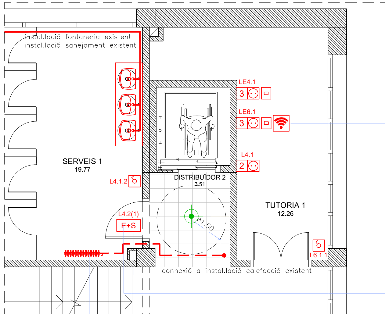
PROPOSTA DISTRIBUCIÓ. PLANTA SEGONA
