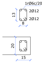
NERVI N1
