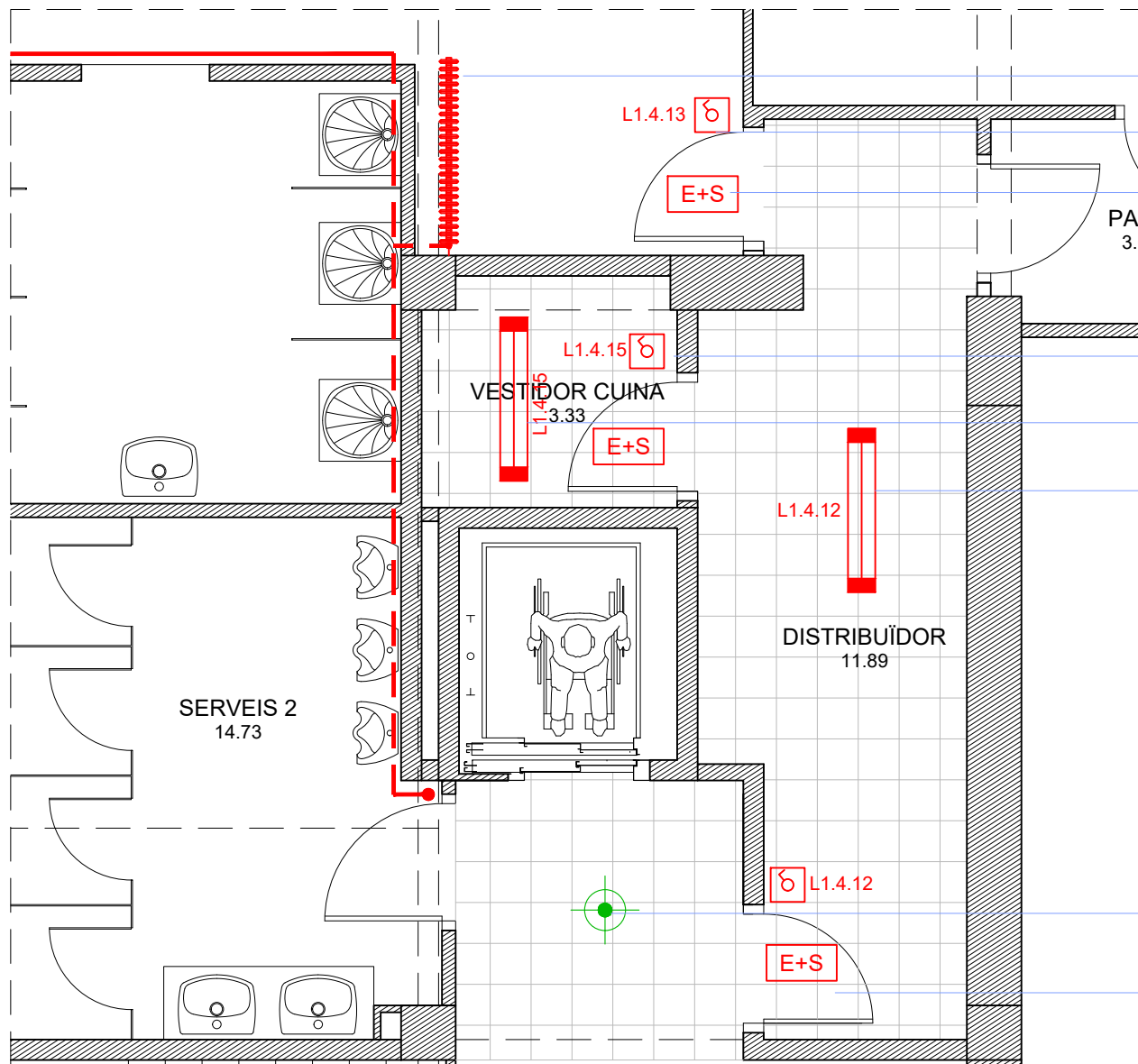
PROPOSTA DISTRIBUCIÓ. PLANTA BAIXA
