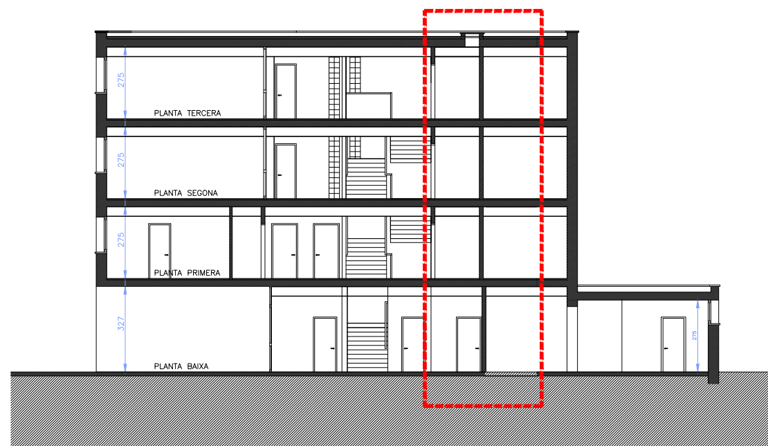
SECCIÓ A-A'
