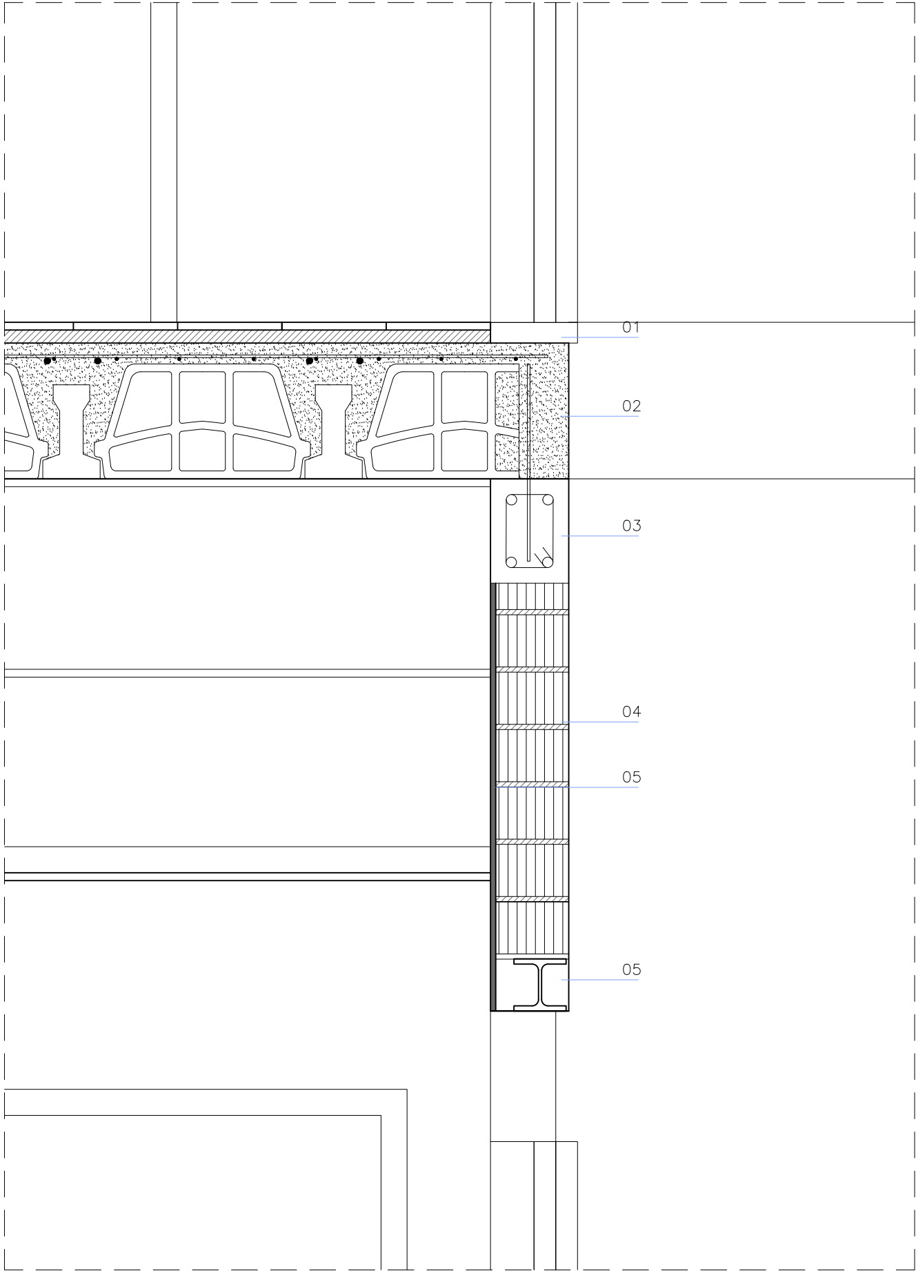
DETALL D02
