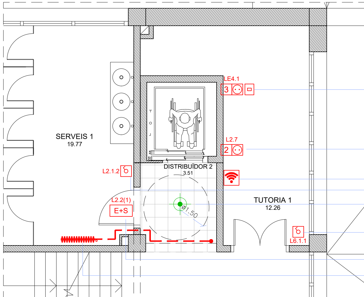
PROPOSTA DISTRIBUCIÓ. PLANTA PRIMERA
