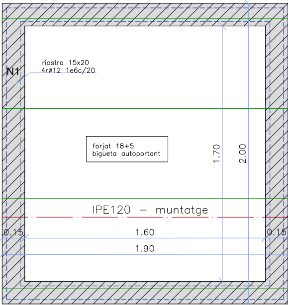
PLANTA COBERTA - D3
