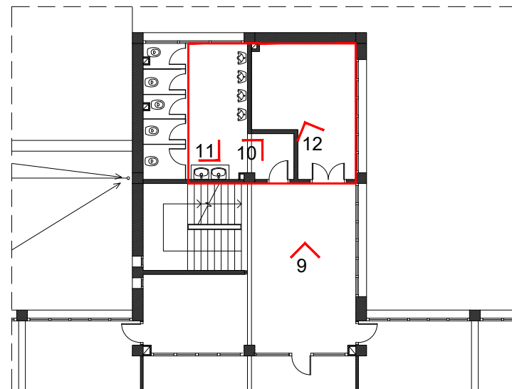
PLANTA SEGONA
