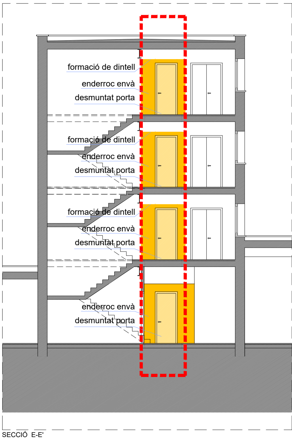
SECCIÓ E-E'
