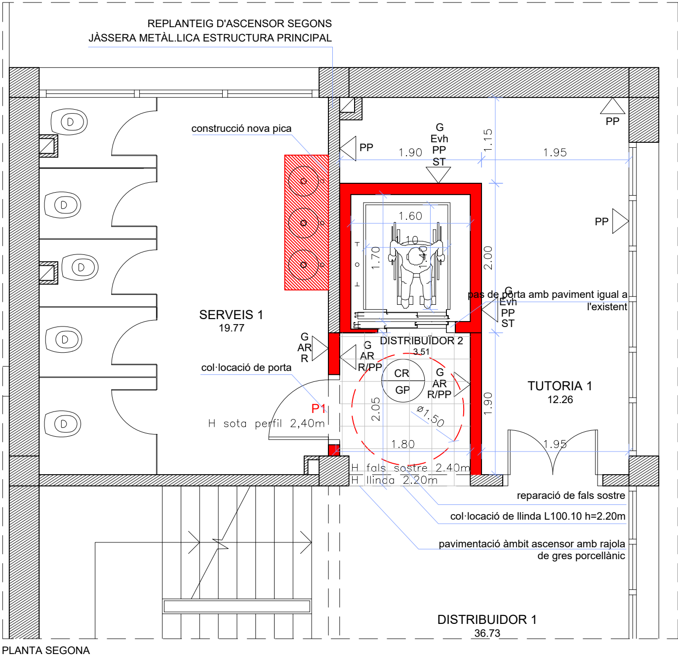
PLANTA SEGONA
