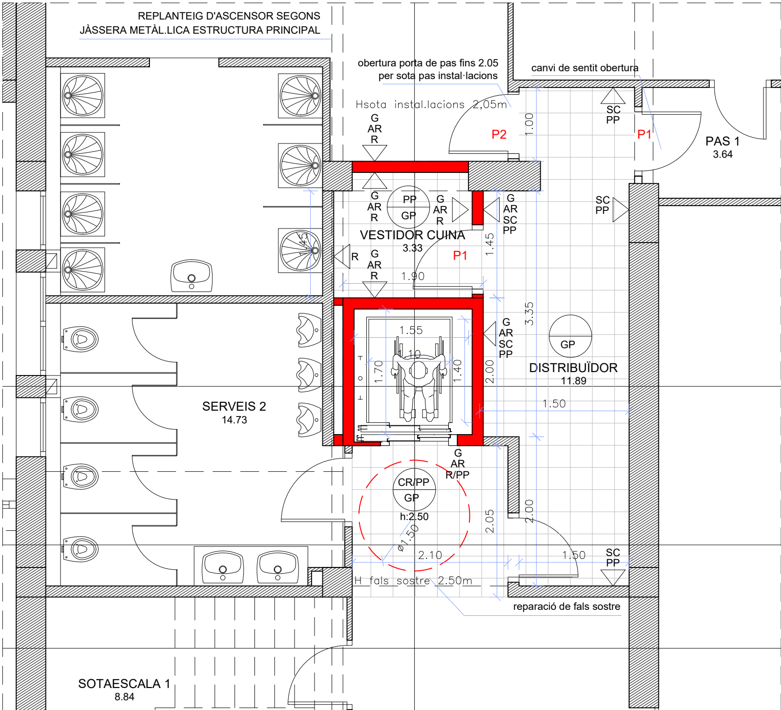
PLANTA BAIXA
