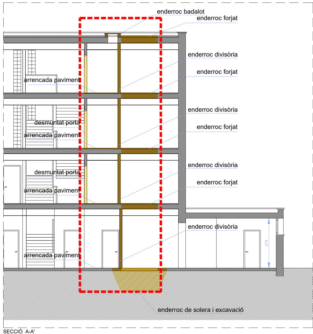
SECCIÓ A-A'
