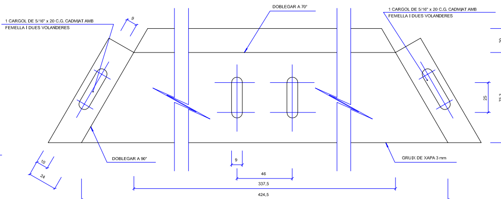
ANCORATGE "B" ESCALA 1:1
