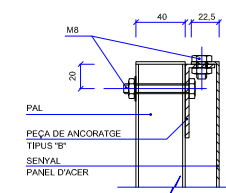
DETALL DE ANCLATGE "A" ESCALA 1:2
