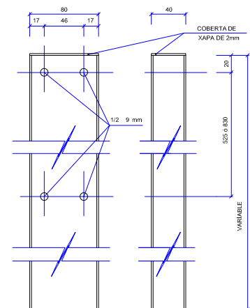
PAL DE SOSTENCIÓ PER A SENYALS ESCALA 1:2
