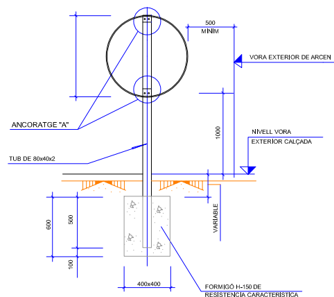
SENYAL CIRCULAR ESCALA 1:20
