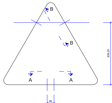
ORIFICIS PER ANCORATGES DE SENYAL TRIANGULAR DE 1350 mm ESCALA 1:5
