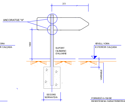
SENYAL DE DIRECCIÓ PROPIA ESCALA 1:20
