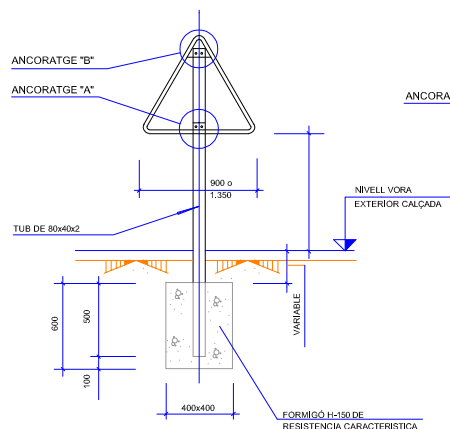
SENYAL TRIANGULAR ESCALA 1:20
