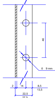
SECCIÓ A-A ESCALA 1:1
