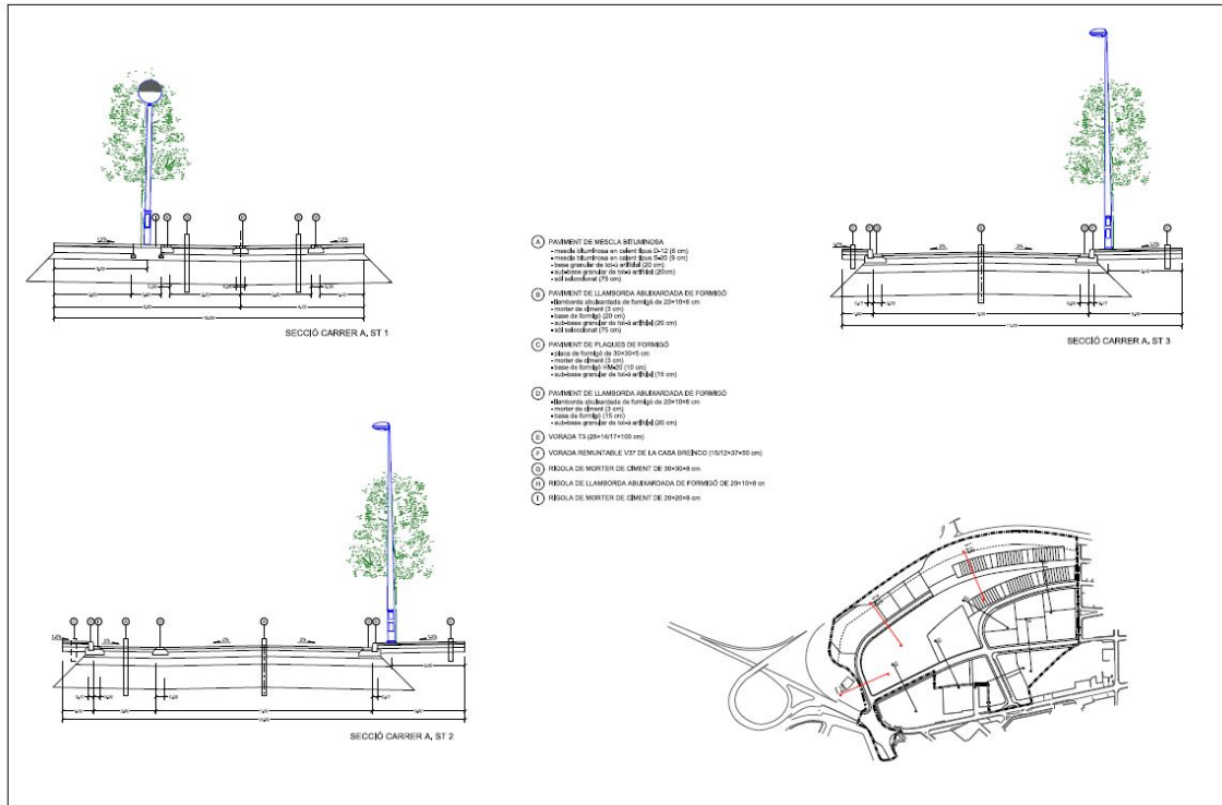
Figura 31. Exemple plànol AAAASOOO_10-Seccions tipus.dgn/dwg
