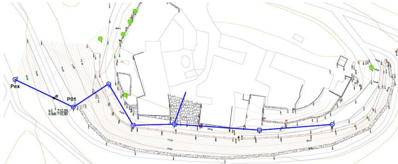
Xarxa de clavegueram existent
