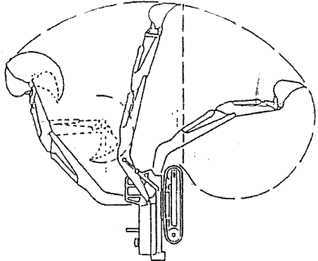
Retroexcavadora
