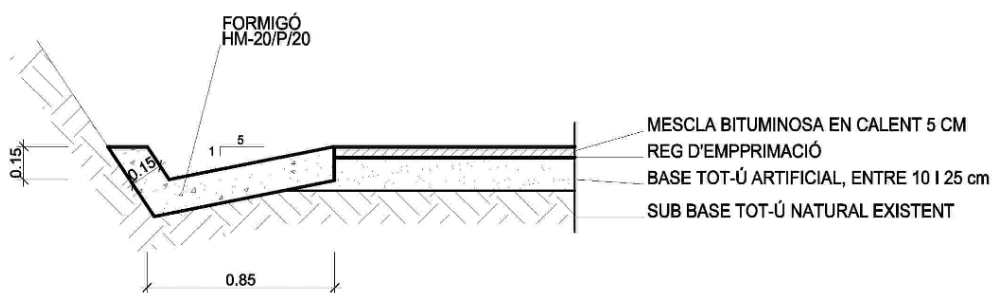
Figura 1. Detall cuneta.
