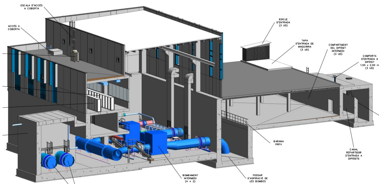
Figura 3. Vista del dipòsit i l'estació de bombament intermedi
