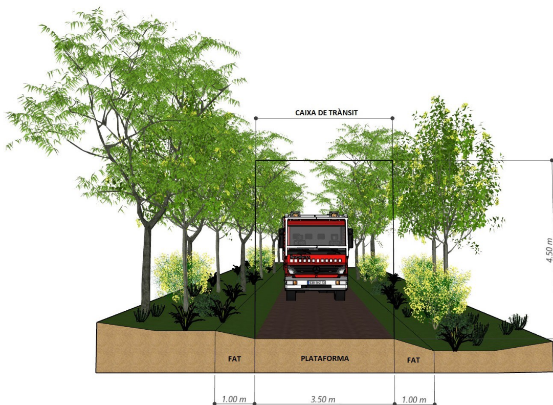
Figura 2. Parts d'un vial de la XVB; plataforma de rodament i FAT (amplades mínimes)
