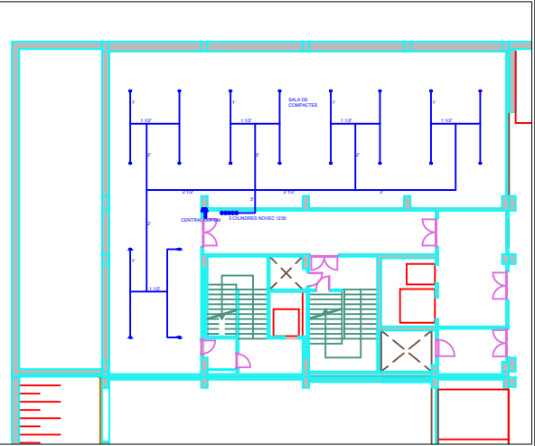
PLANTA SOTERRANI
