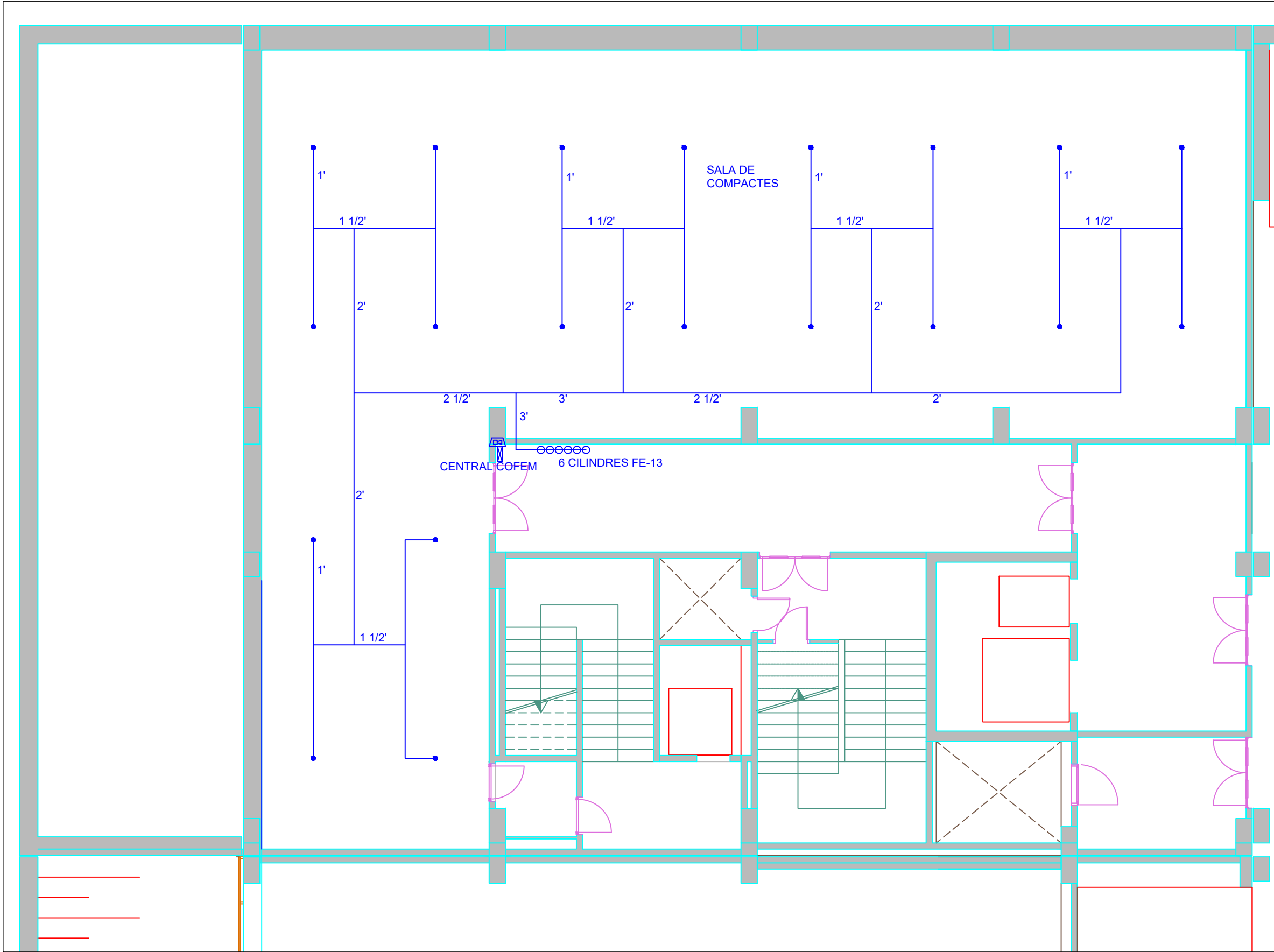
PLANTA SOTERRANI
