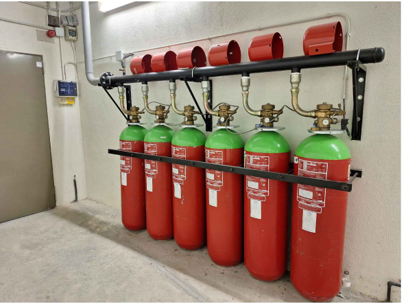
6 CILINDRES FE-13
