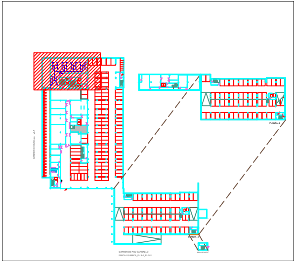
PLANTA SOTERRANI
