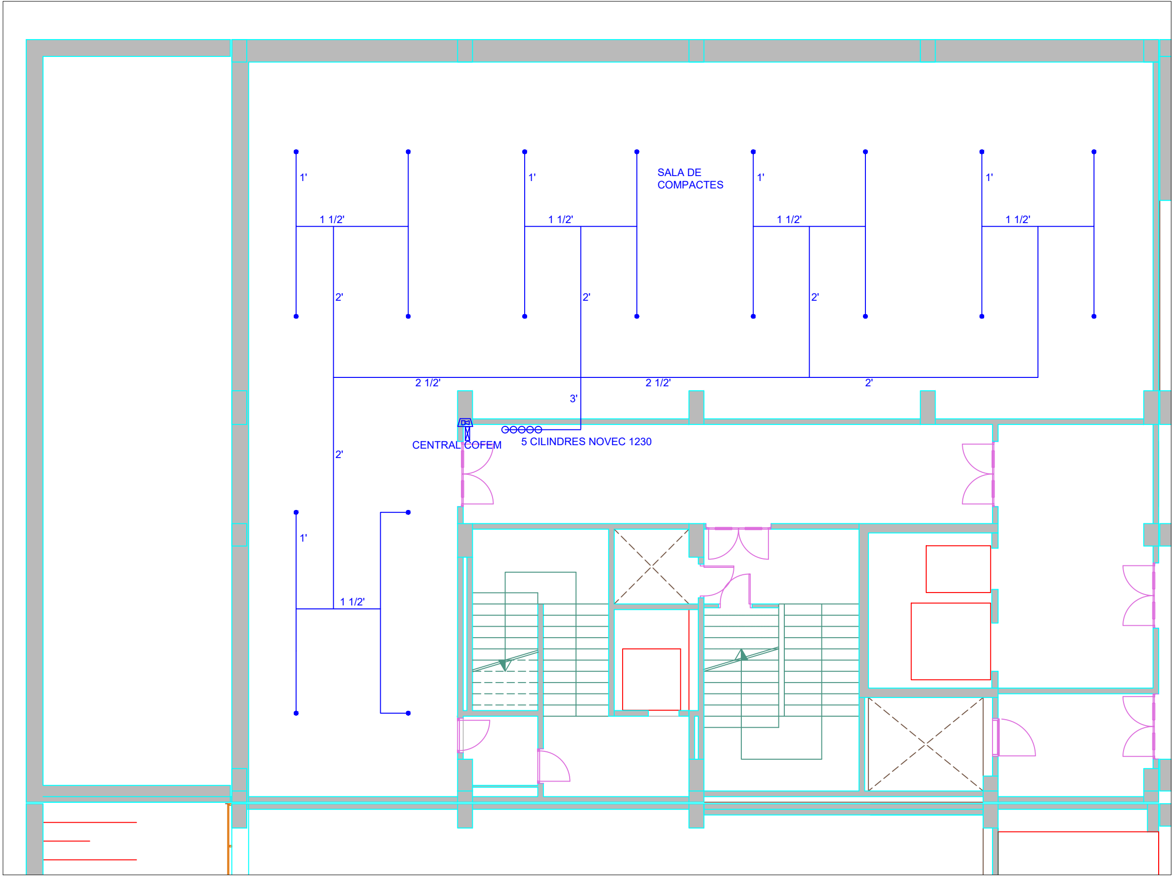
PLANTA SOTERRANI
