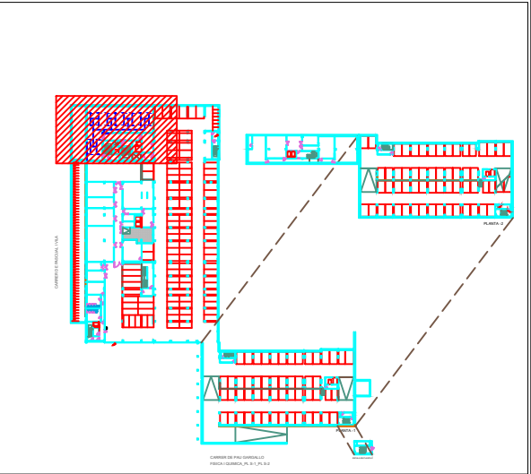
PLANTA SOTERRANI
