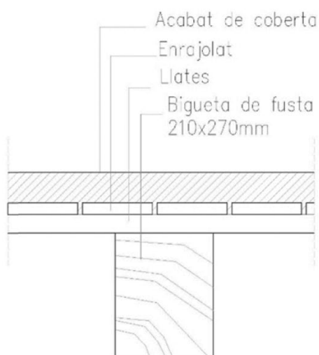
Forjat de coberta: tauler ceràmic sobre llantes de fusta
