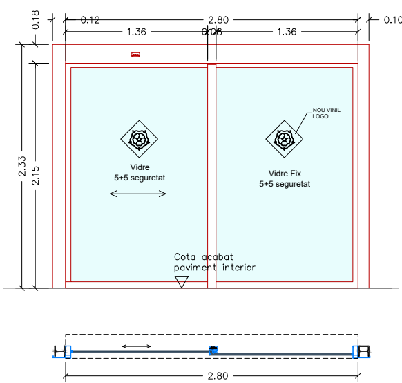
Porta automàtica de dues fulles, comprovació de mides a l'obra, amb obertura lateral dreta o esquerra, amb perfil biga. Fulla fixa i fulla corredissa, amb vidre laminat de seguretat transparent 5+5. Inclou pany i clau, així com la subestructura necessària per a la seva correcta instal·lació. Vinil amb cairó del logotip de l'Ajuntament de Reus. 1 unitat
