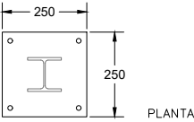
DETALL PLETINES ANCLATGE A TERRA DELS PILARS HEB 100 250x250x12mm i perns 4 Ø 12
