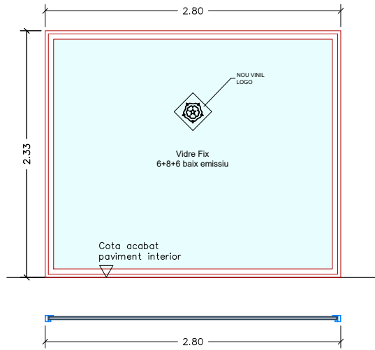
Finestral fix d'alumini, amb trencament de pont tèrmic, acabat lacat RAL color i mides a definir a l'obra. Vidre fix baix emissiu 6+8+6mm. Vinil amb cairó del logotip de l'Ajuntament de Reus. 1 unitat
