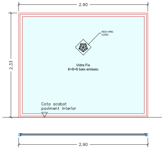
Finestral fix d'alumini, amb trencament de pont tèrmic, acabat lacat RAL color i mides a definir a l'obra. Vidre fix baix emissiu 6+8+6mm. Vinil amb cairó del logotip de l'Ajuntament de Reus. 1 unitat
