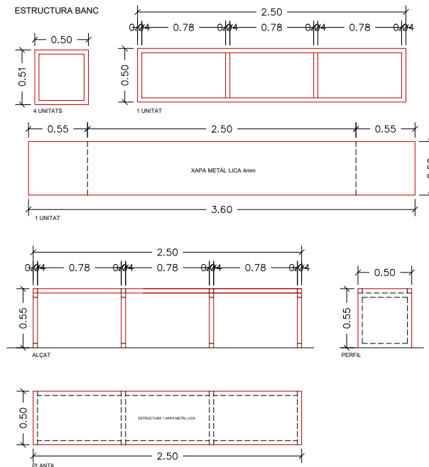
Banc de perfils metàl·lics 40x40mm i xapa metàl·lica 4mm pintada, color a definir a l'obra. 1 unitat
