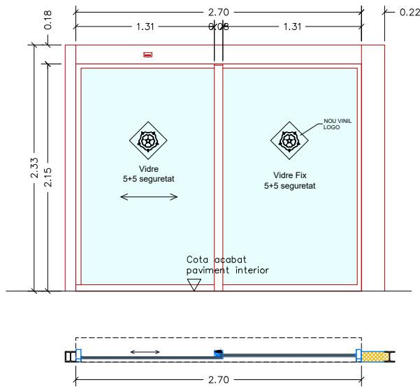
Porta automàtica de dues fulles, comprovació de mides a l'obra, amb obertura lateral dreta o esquerra, amb perfil biga. Fulla fixa i fulla corredissa, amb vidre laminat de seguretat transparent 5+5. Inclou pany i clau, així com la subestructura necessària per a la seva correcta instal·lació. Vinil amb cairó del logotip de l'Ajuntament de Reus. 1 unitat
