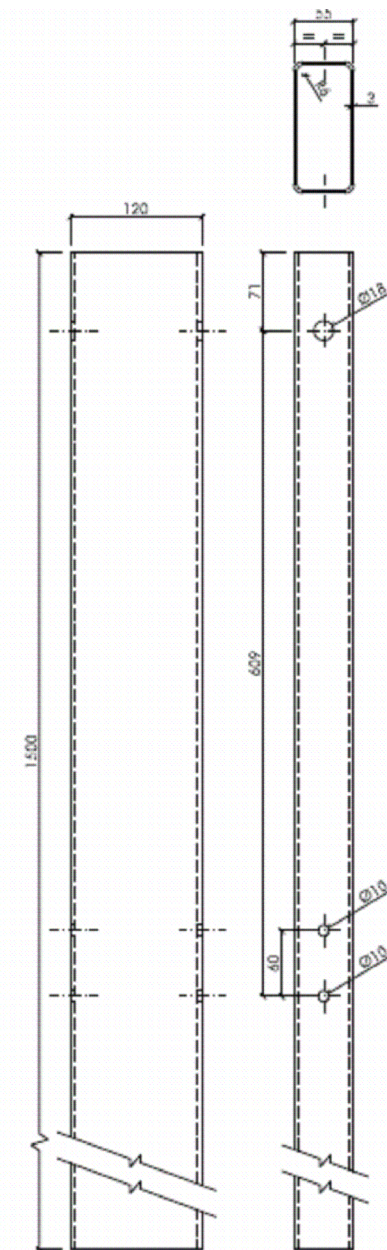
POSTE TUBULAR 1,5m. ESCALA 1:5
