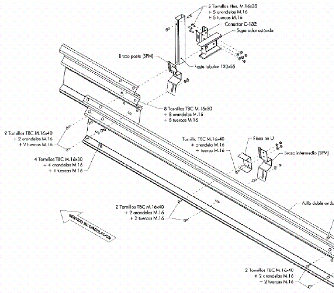
ISOMÉTRICA FRONTAL Escala 1:10
