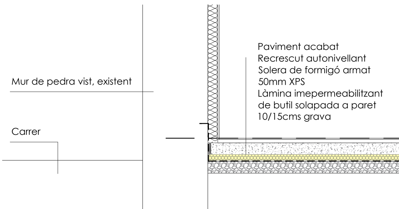
Detall Base mur existent / paviment interior
