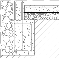
DETALLE ZAPATA, MURO Y SOLERA
