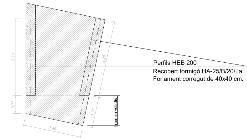
LLOSA FORMIGÓ RECOLZADA SOBRE PERFILS HEB 200
