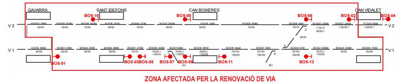
Figura 11 Elements del sistema de senyalització a via controlats per l'enclavament de Can Boixeres.
