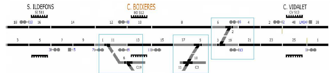
Figura 14 Accionaments d'agulla en la zona de Can Boixeres.
