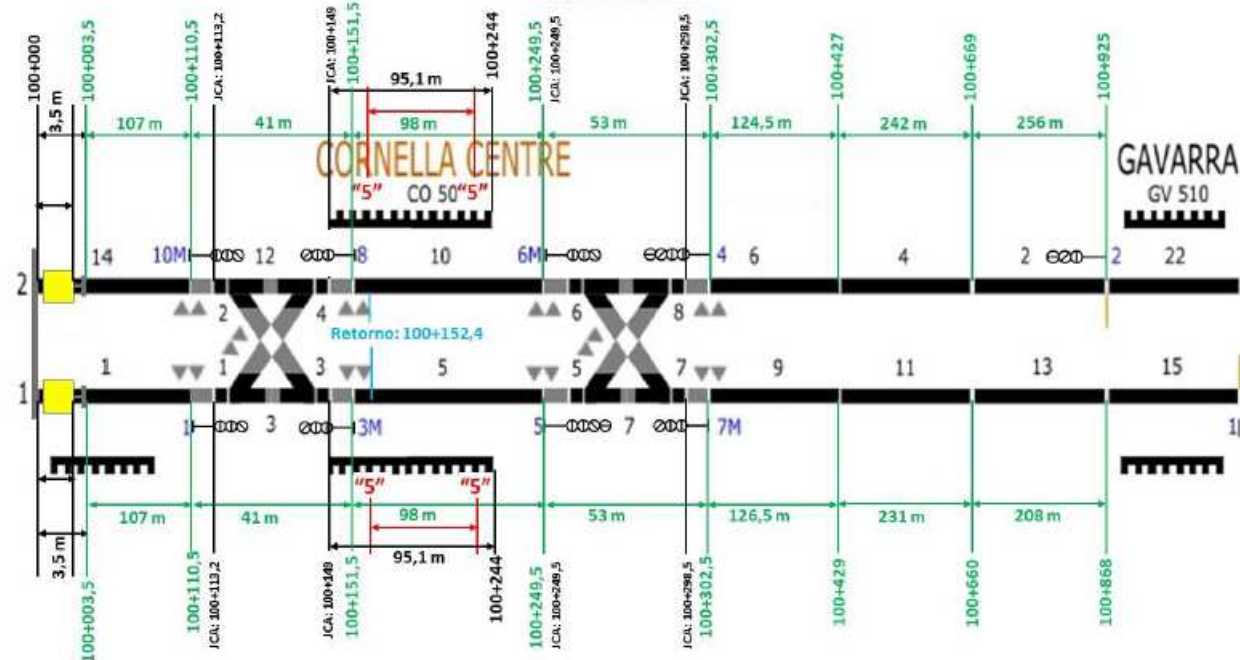
Figura 5 Esquema de detall de la cua de maniobra de Cornellà Centre amb les Bretelles.
