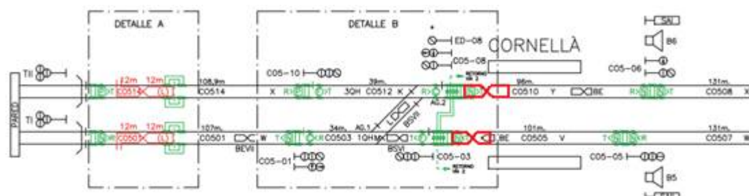
Figura 10 Nous llaços d'emergència a Cornellà Centre.
