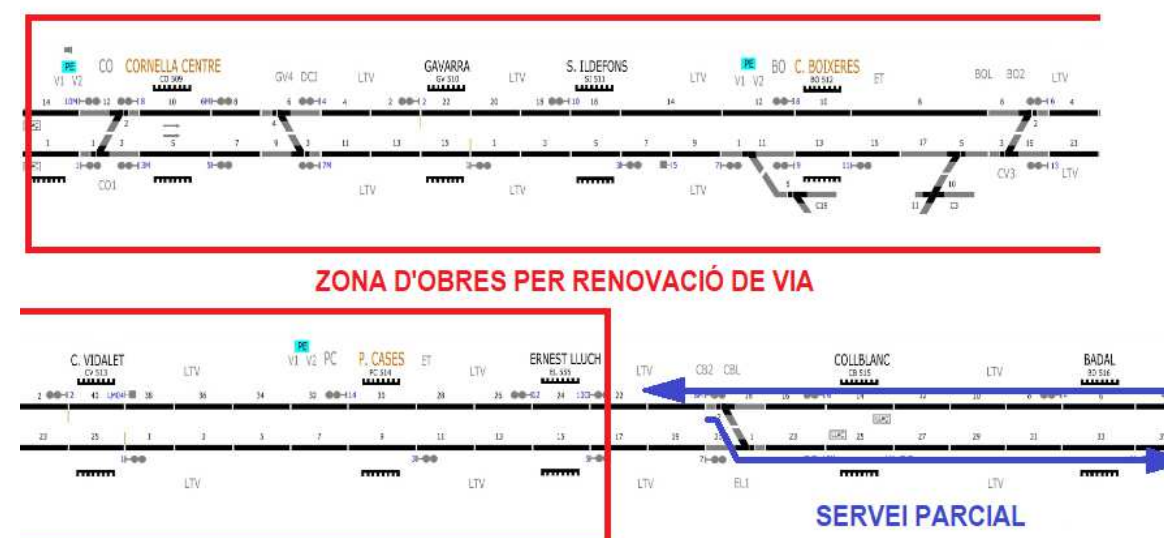
Figura 3 Zona en vermell afectada per la renovació de via.
