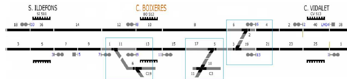
Figura 6 Accionaments d'agulla en la zona de Can Boixeres.
