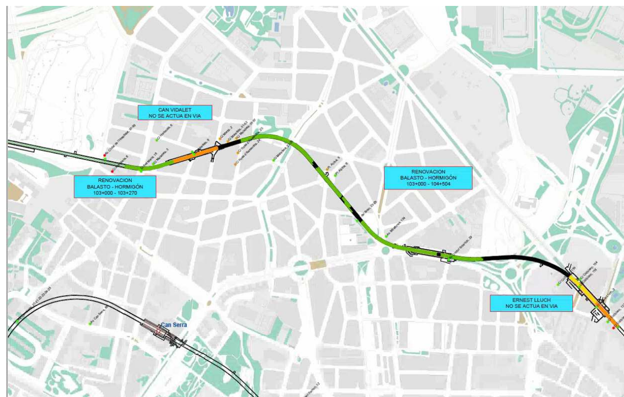
Figura 2 Renovació de via entre Can Vidalet i Ernest Lluch L5 FMB.
