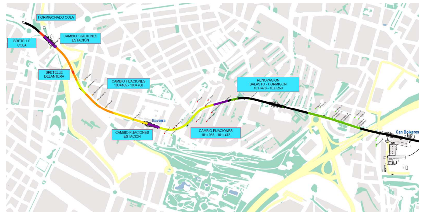
Figura 1 Renovació de via entre Cornellà Centre i Can Boixeres L5 FMB.
