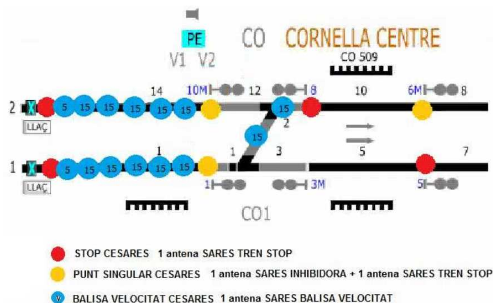
Figura 5 Tipologies de conjunts Train Stop al fons de maniobra de Cornellà Centre.
