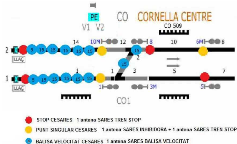
Figura 13 Tipologies de conjunts Train Stop al fons de maniobra de Cornellà Centre.
