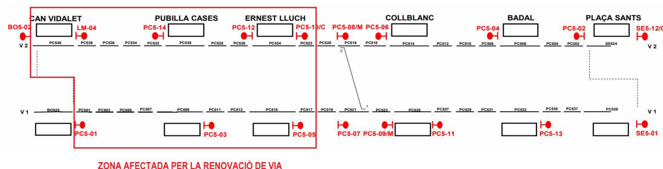
Figura 12 Elements del sistema de senyalització a via controlats per l'enclavament de Pubilla Cases.
