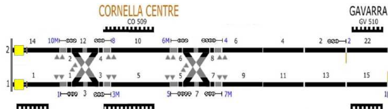
Figura 4 Esquema del cul de sac de Cornellà Centre amb l'obra finalitzada.
