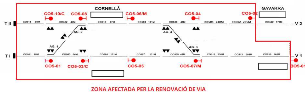
Figura 9 Elements del sistema de senyalització a via controlats per l'enclavament de Cornellà Centre.
