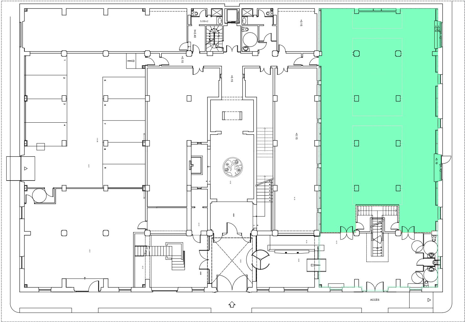
PLANTA BAIXA
