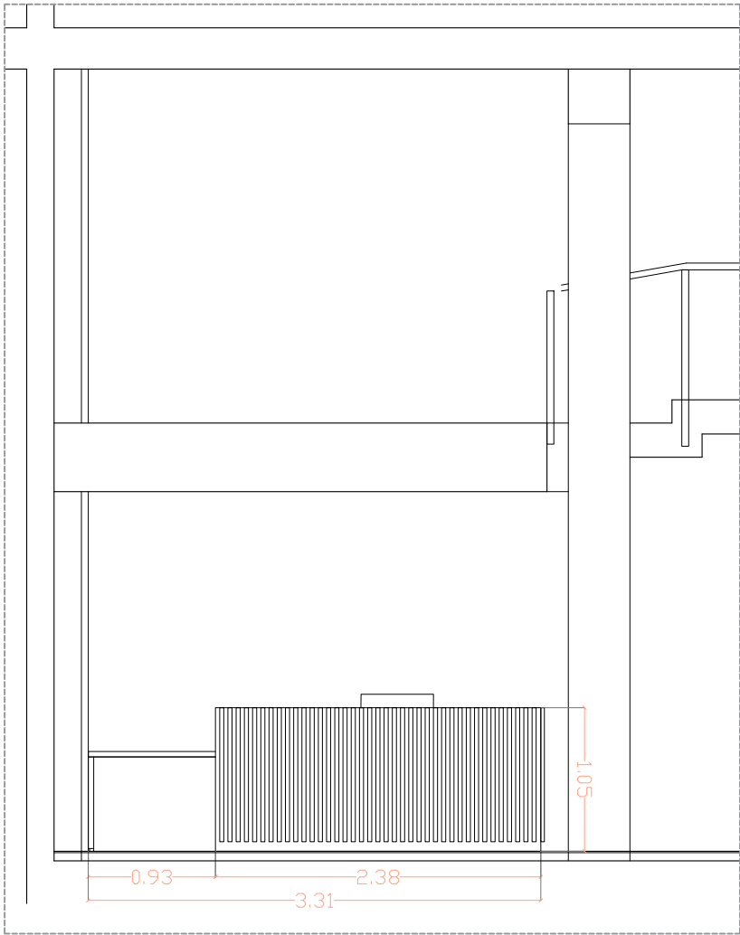
ALÇAT MOSTRADOR DES DE L'ENTRADA
