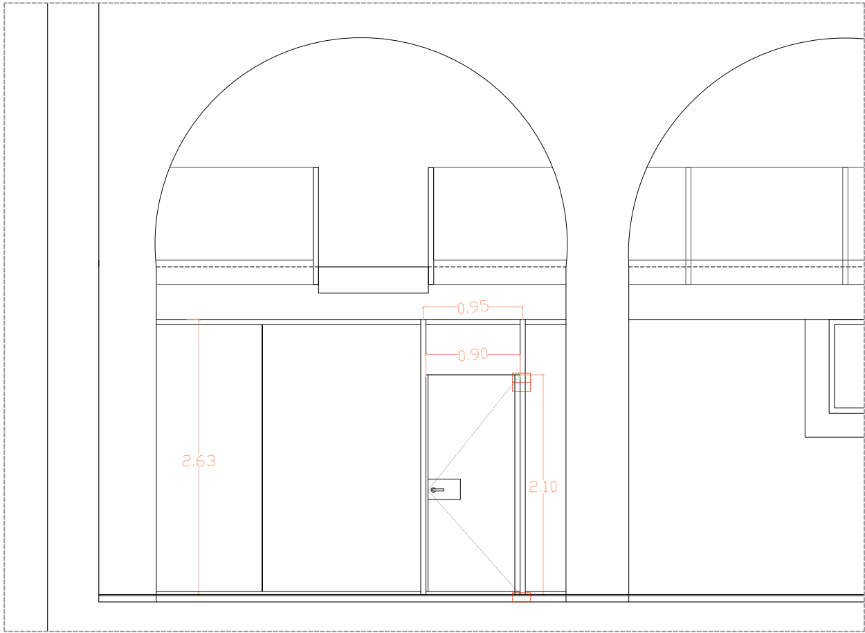
ALÇAT DETALL
