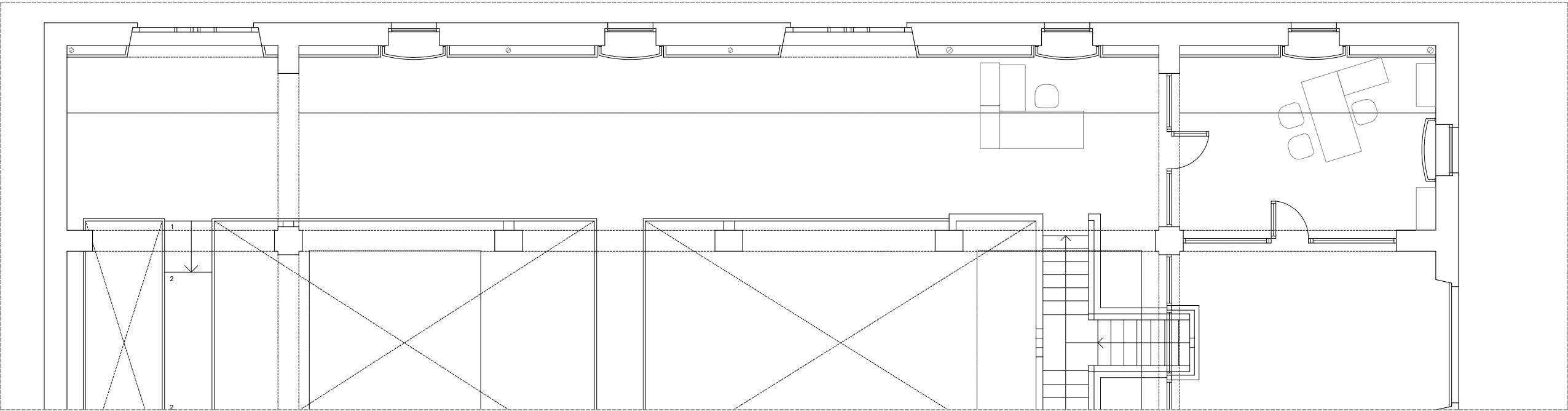
PLANTA ENTRESOL
