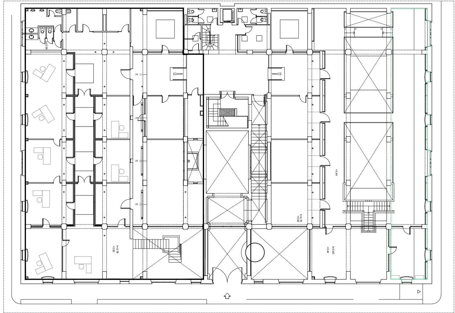
PLANTA ENTRESOL
