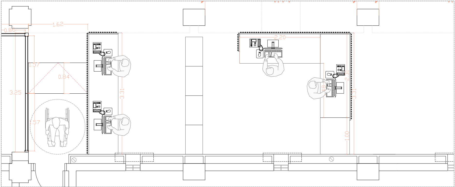
PLANTA DETALL ZONA AUTOSERVEI I MOSTRADOR D'ACCÉS
