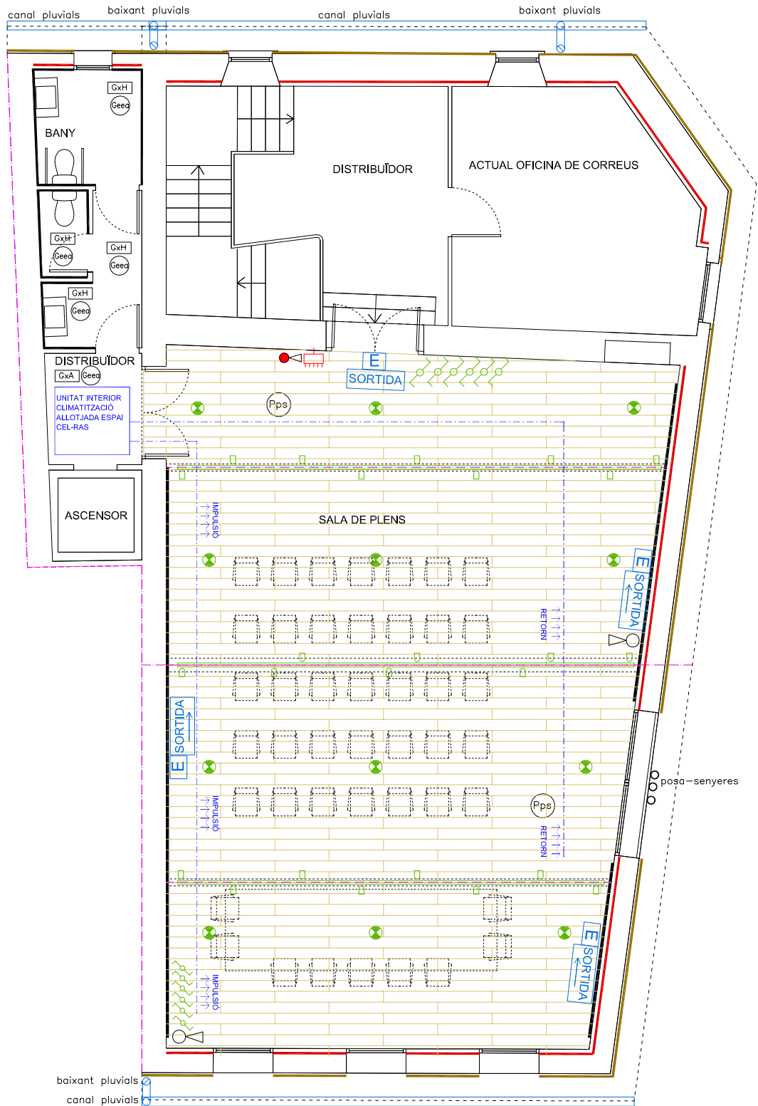
PLANTA SEGONA
