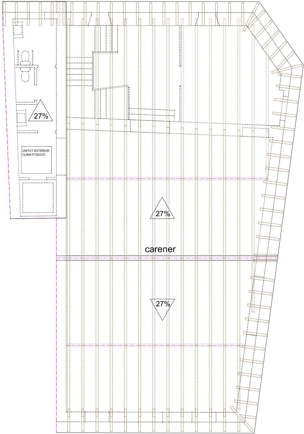
PLANTA COBERTA
