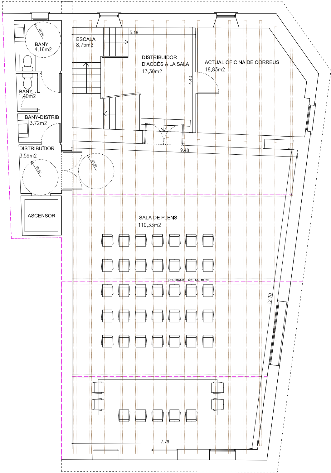
PLANTA SEGONA
