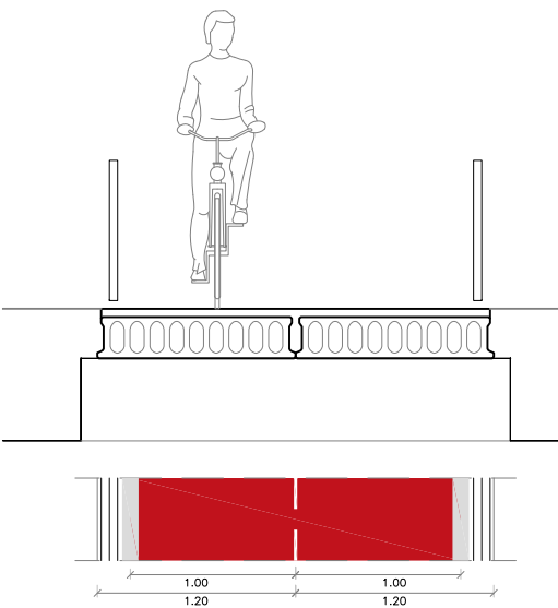
SECCIÓ TRANSVERSAL (E:1/50)
