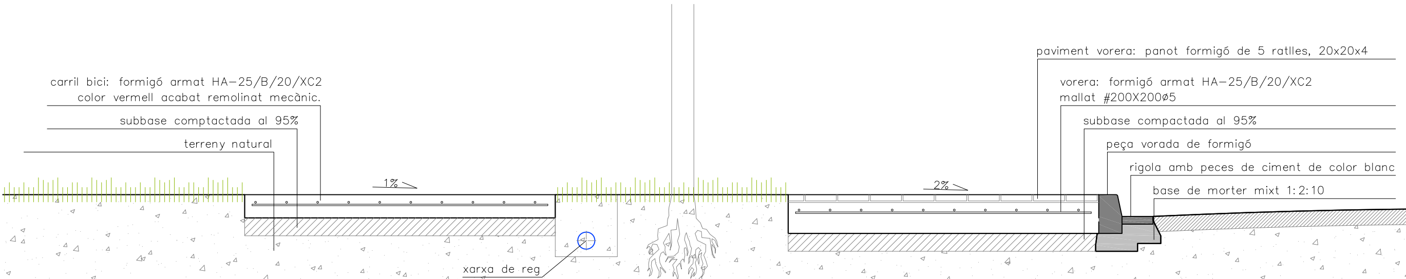
SECCIÓ TIPUS CARRIL BICI I VORERA (E:1/25)
