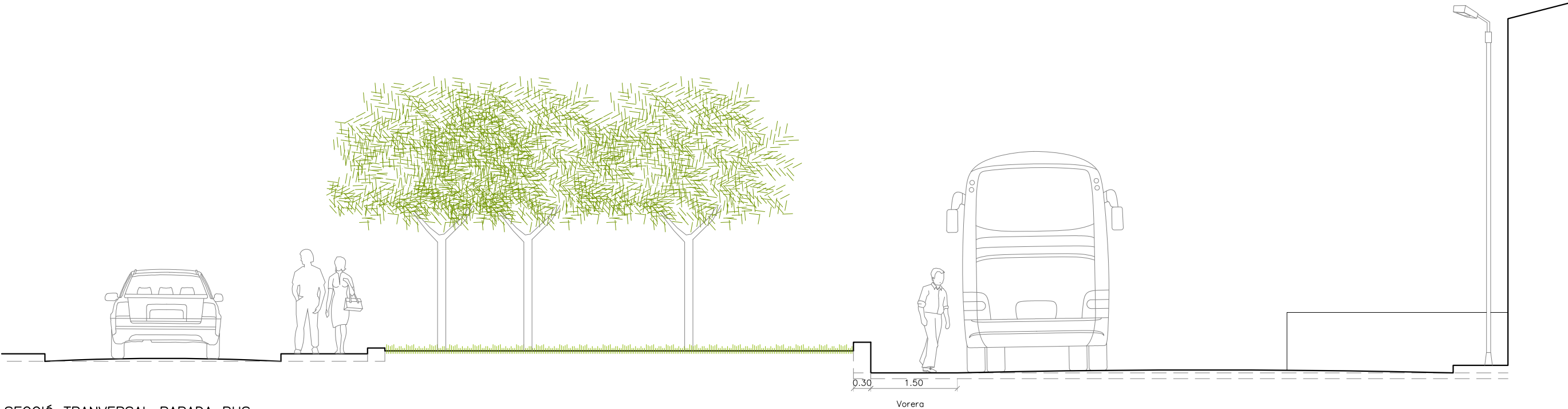
SECCIÓ TRANSVERSAL PARADA BUS
