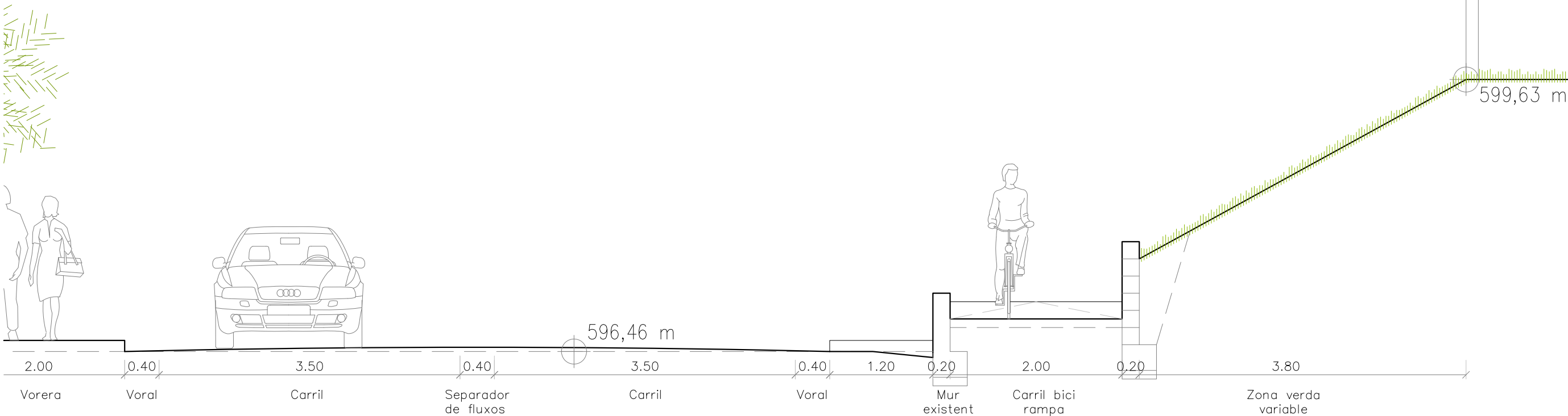
SECCIÓ TRANSVERSAL B-B' (E:1/50)
