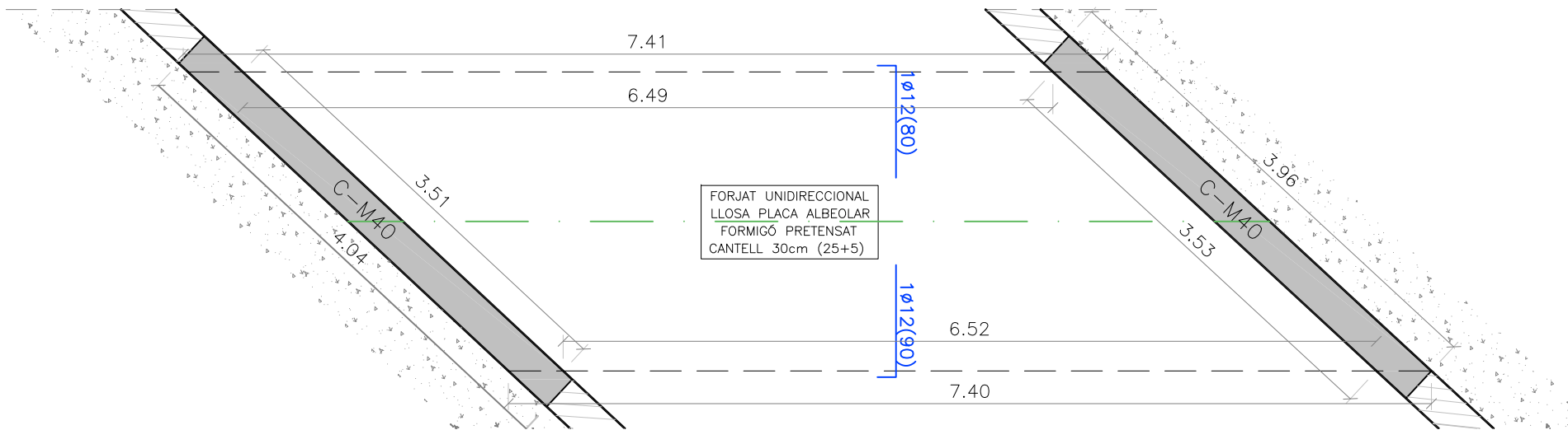
SECCIÓ LONGITUDINAL (E:1/50)
