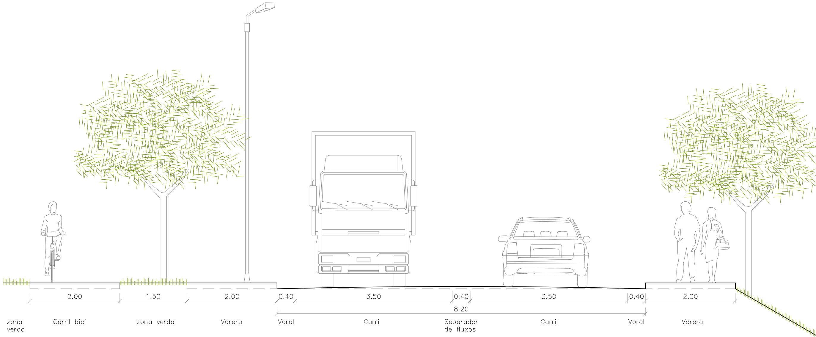
SECCIÓ TIPUS CARRETERA C-12.
