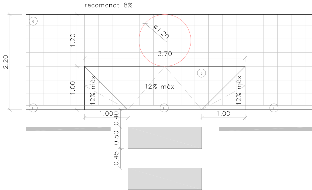
GUAL DE TRES RAMPES I PAS DE VIANANTS. (E:1/50) PLANTA TIPUS
