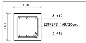
CERCOL C-M40
