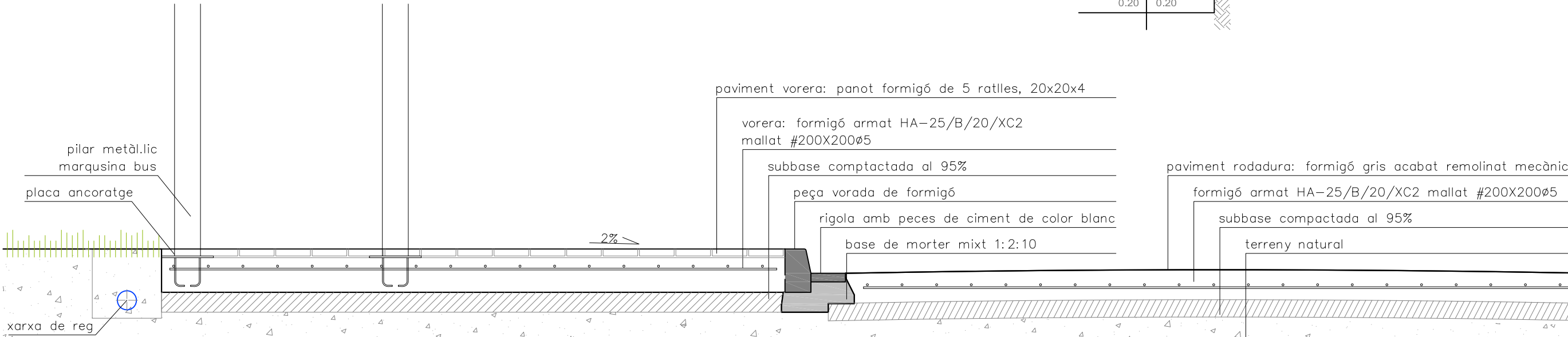
SECCIÓ TRANSVERSAL NOVA PARADA BUS LLEIDA (E:1/25)
