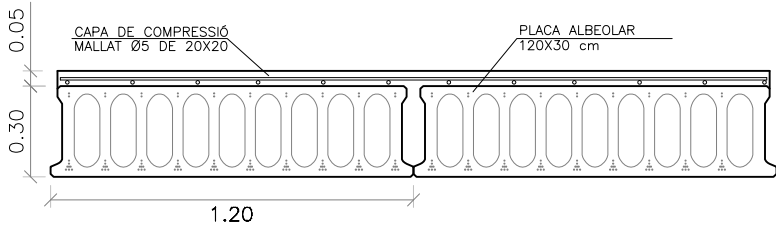
DETALLS CONSTRUCTIUS (E:1/25)
