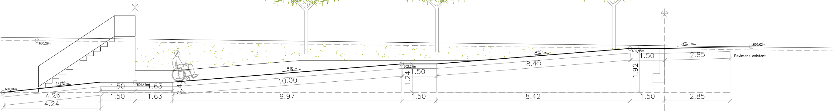
SECCIÓ LONGITUDINAL
