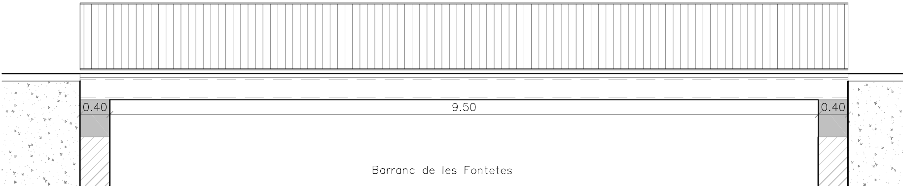
SECCIÓ LONGITUDINAL (E:1/50)
