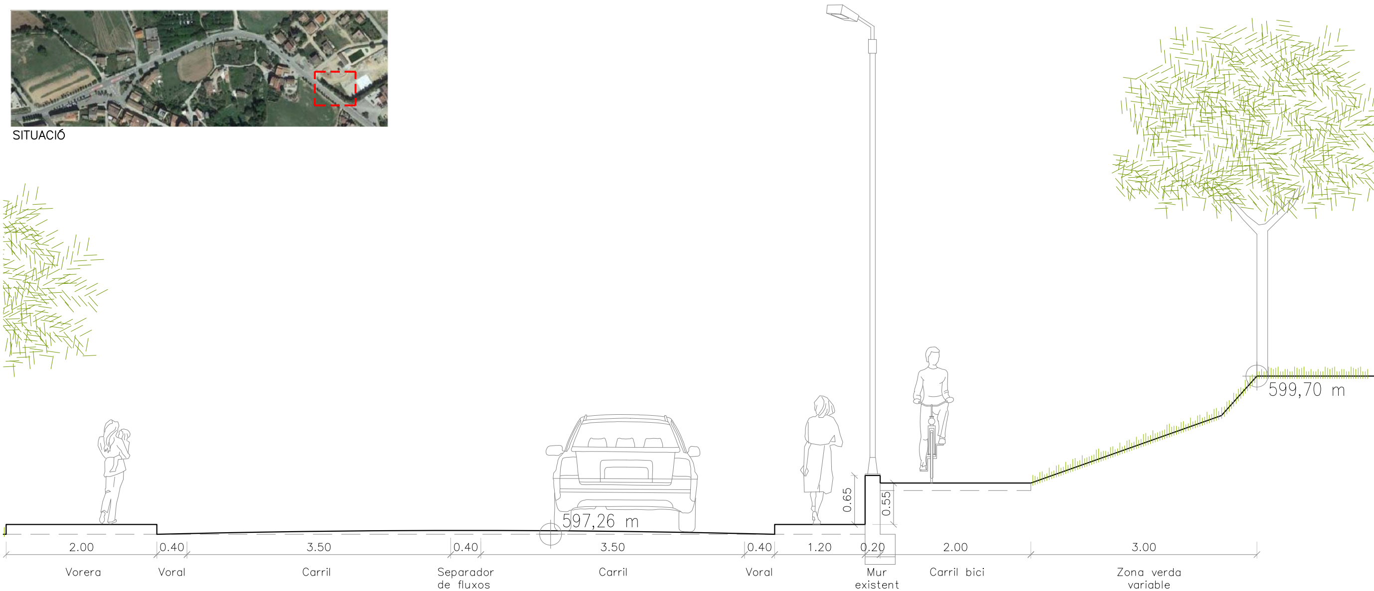
SECCIÓ TRANSVERSAL A-A' (E:1/50)
