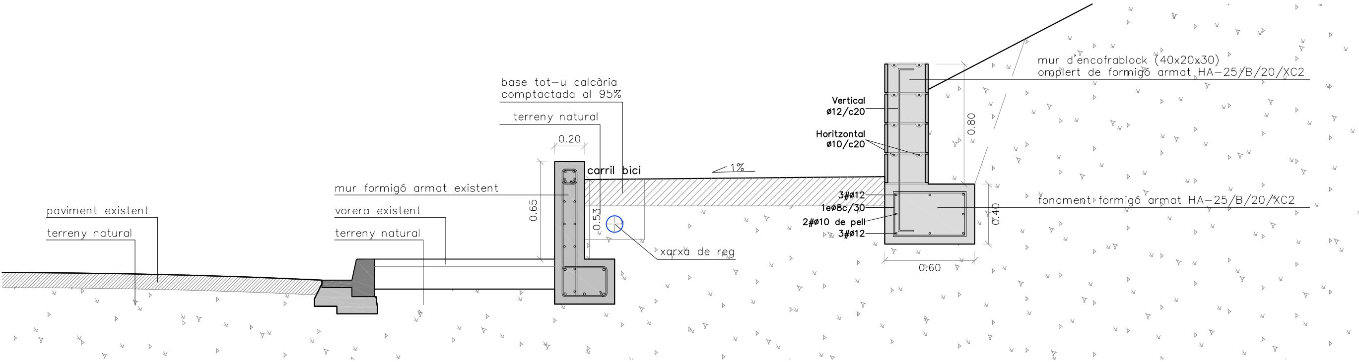
SECCIÓ TRANSVERSAL (E:1/25)
