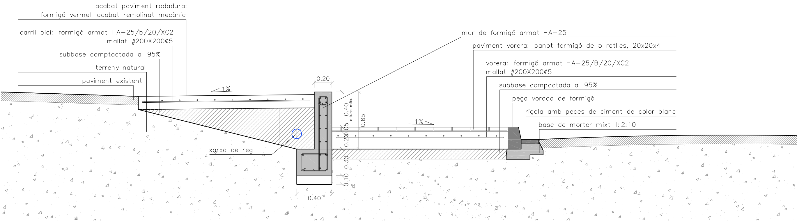
SECCIÓ TRANSVERSAL VORERA-MUR-CARRIL BICI (E:1/25)
