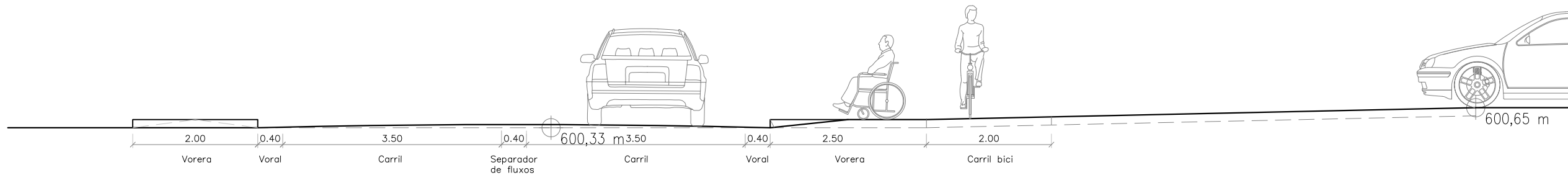
SECCIÓ TRANVERSAL A-A' (E:1/75)
