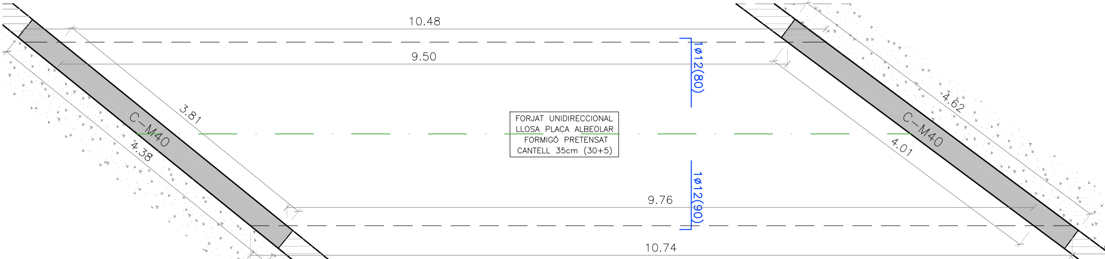
SECCIÓ LONGITUDINAL (E:1/50)
