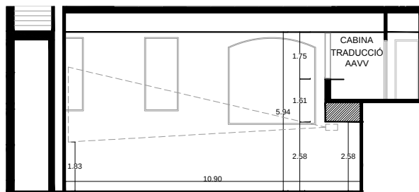
SECCIÓ SALA RAVAL
