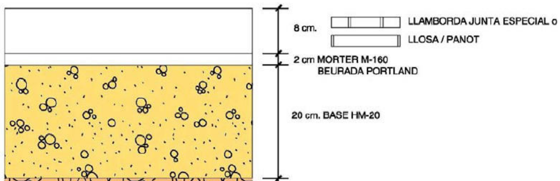
Imatge 39. Paviment del reductor de velocitat amb pas de vianants
