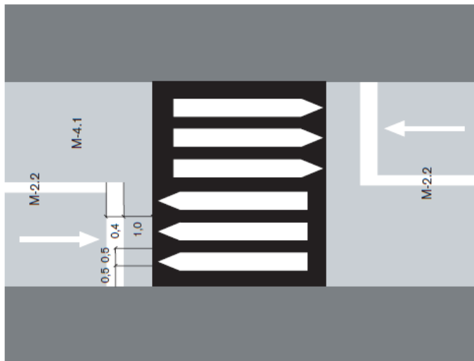
Imatge 40. Senyalització horitzontal dels reductors de velocitat
