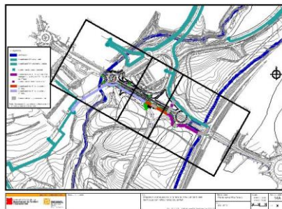
Figura 25. Exemple plànol amb diversos fulls AAAASOOO_14A-Planta MT.dgn/dwg
