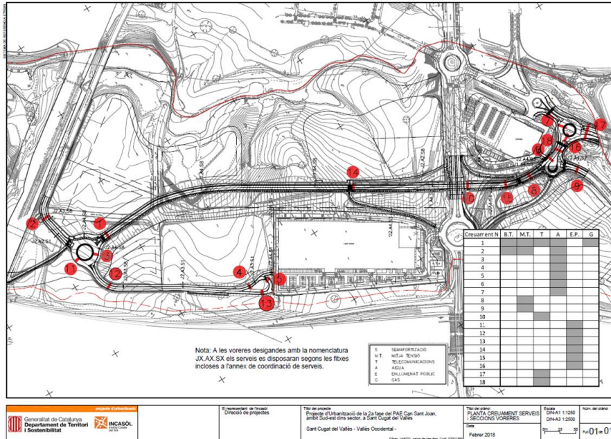
Figura 39. Exemple plànol AAAASOOO_20C-Seccions orientatives.dgn/dwg
