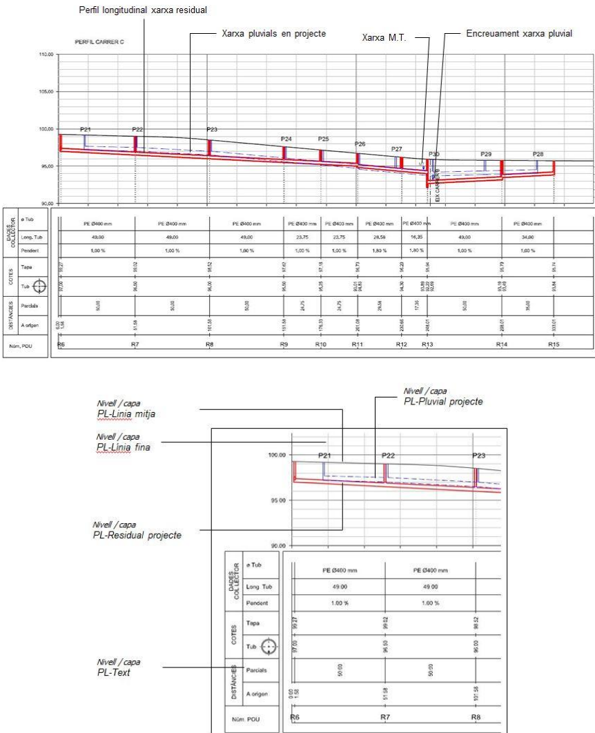
Figura 27. Exemple dels elements a dibuixar a l'espai model de l'arxiu AAAASOOO-12B-Perfils residuals.dgn/dwg
