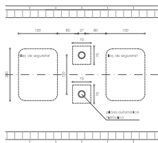
PLANTA T'CHES AUTOMÀTIQUES E. 1/20
