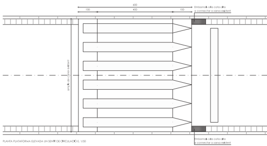
PLANTA PLATFÒRMA ELEVADA UN SENT DE CIRCULACIÓ E. 1/20
