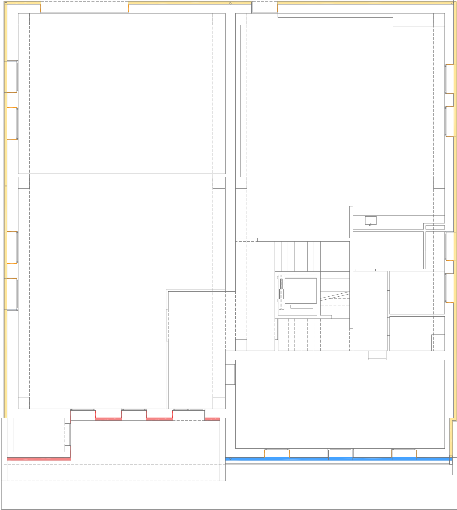
PROPOSTA PLANTA BAIXA
