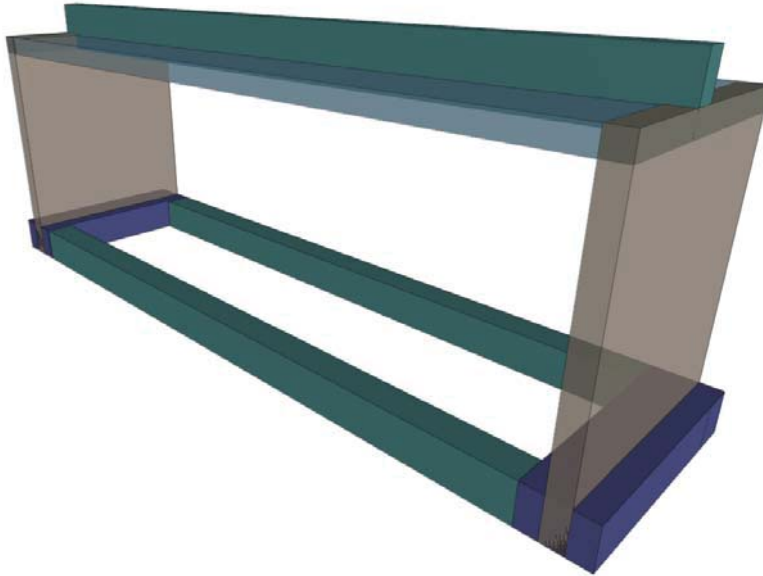
Esquema 3D de l'accés proposat en l'edifici, amb dos sabates corregudes, amb dos riestres que les uneixen, dos pantalles de formigó armat i una llosa superior amb un nervi superior.
