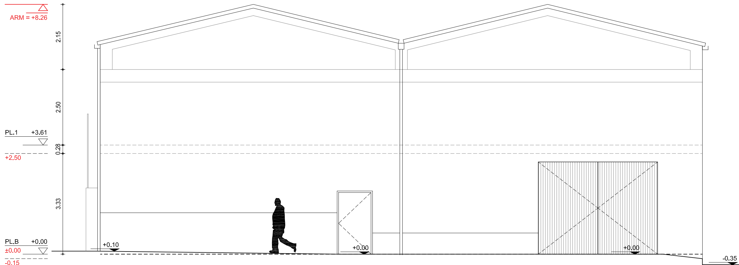
FAÇANA POSTERIOR. NORD
