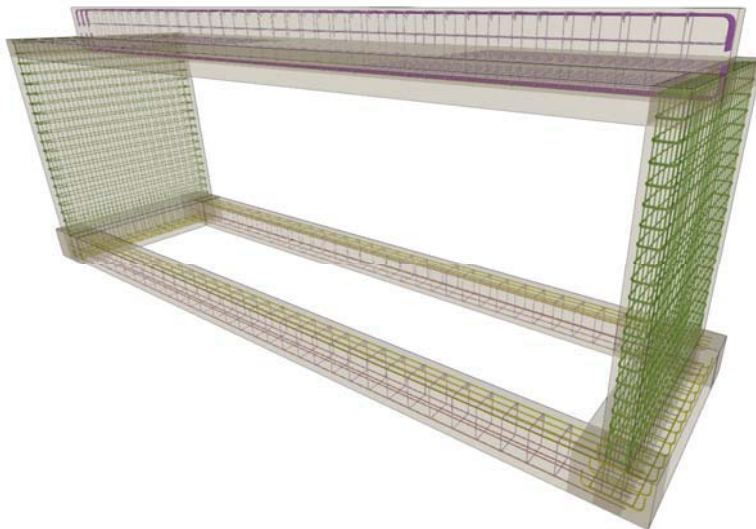
Esquema 3D amb l'armat proposat de l'accés proposat en l'edifici, amb dos sabates corregudes, amb dos riestres que les uneixen, dos pantalles de formigó armat i una llosa superior amb un nervi superior.
