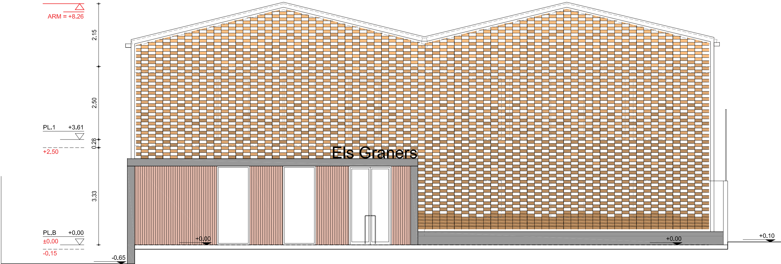
FAÇANA DAVANT. SUD
