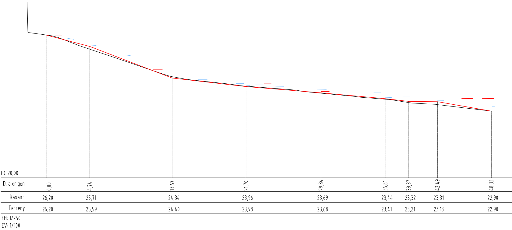
C/DE LA PAU. RASANT DE PROJECTE
