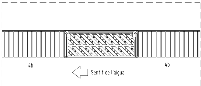
RIGOLA TIPUS
