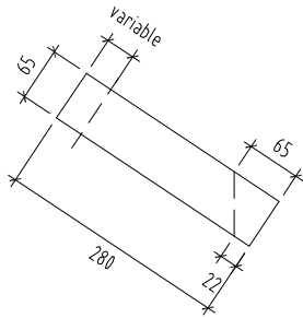
PAVIMENT INCLINAT BASE
