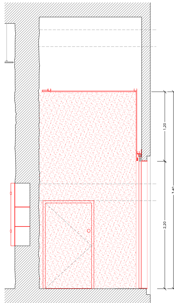
ALÇAT E-E'
