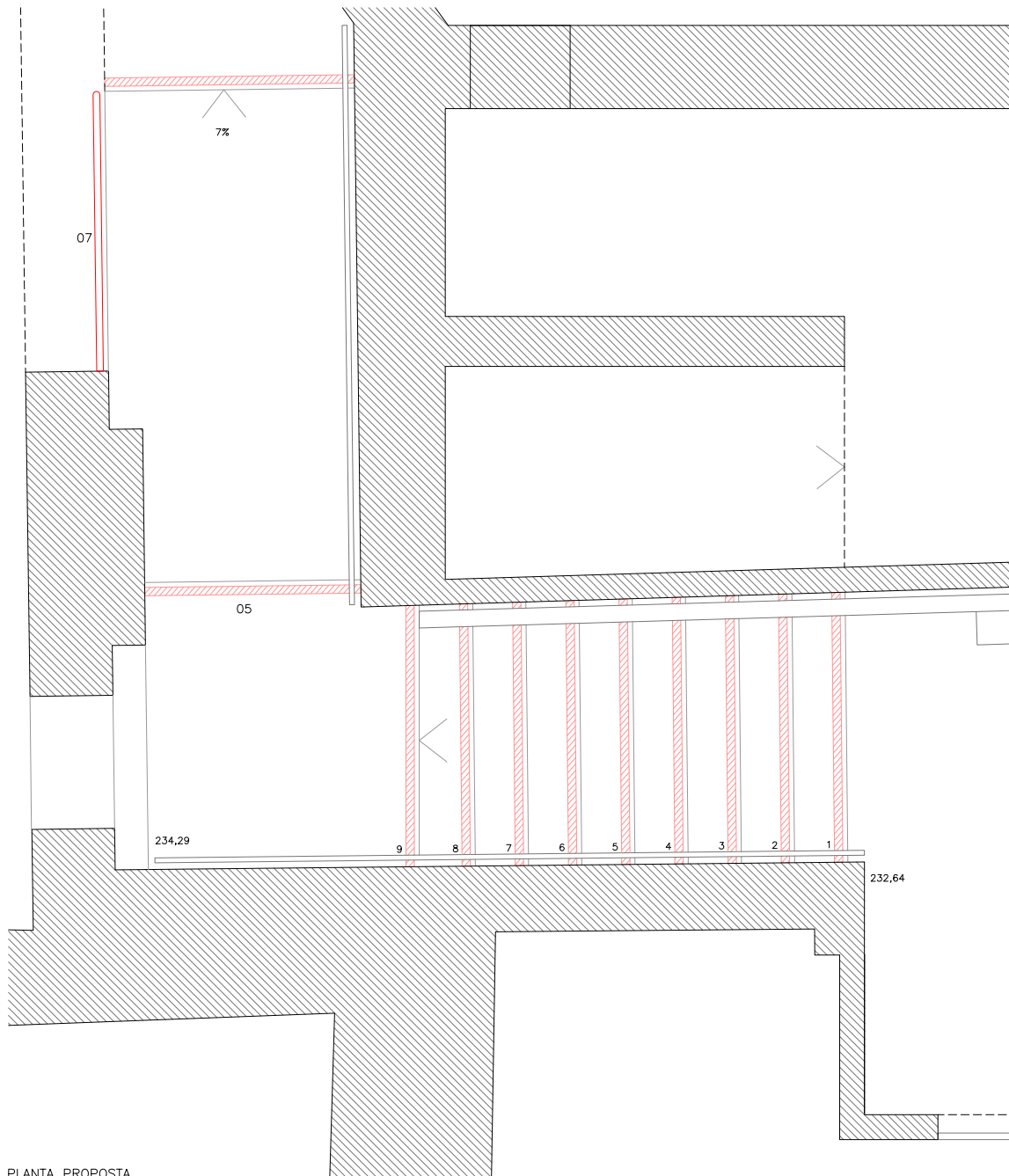
PLANTA PROPOSTA
