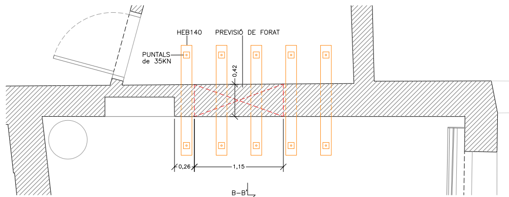
PLANTA ESTINTOLAMENT PROVISIONAL
