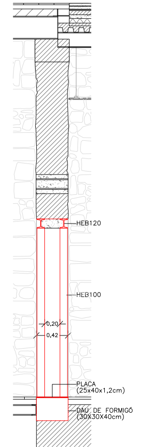
SECCIÓ B-B'
