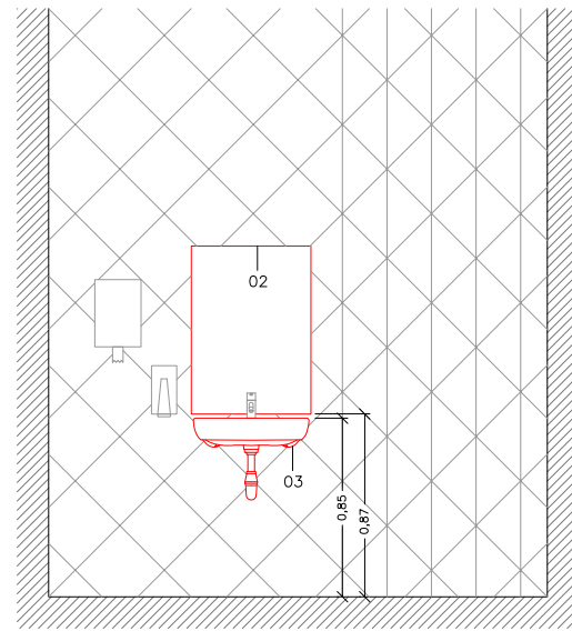
ALÇAT A-A' (PROPOSTA)
