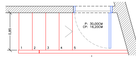
PLANTA PROJECTE (FASE II)
