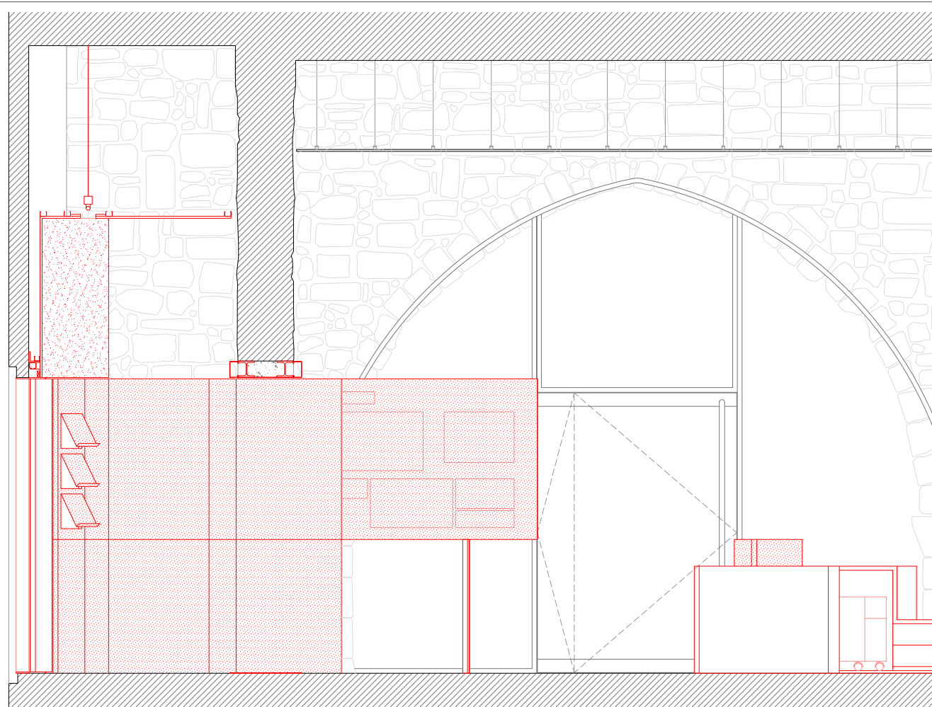
ALÇAT C-C'
