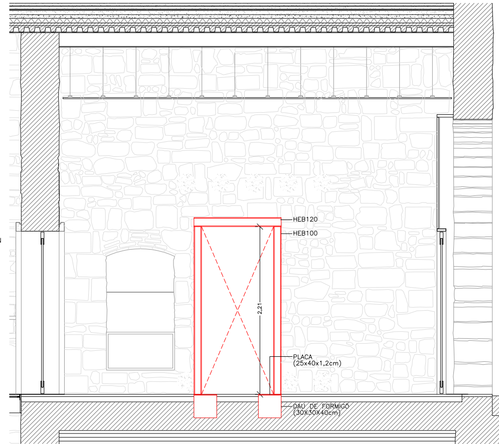
ALÇAT A-A' PÒRTIC
