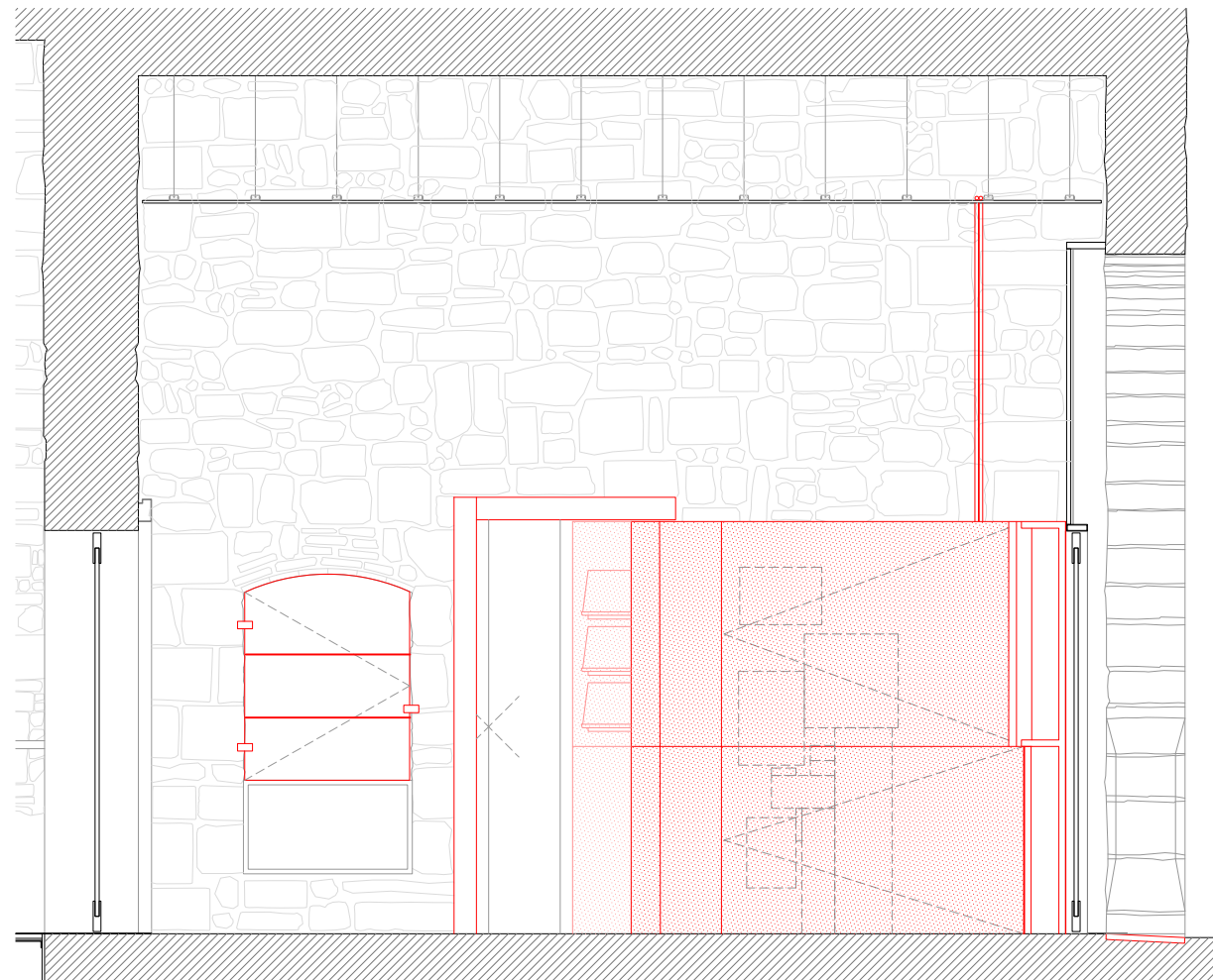
ALÇAT D-D'
