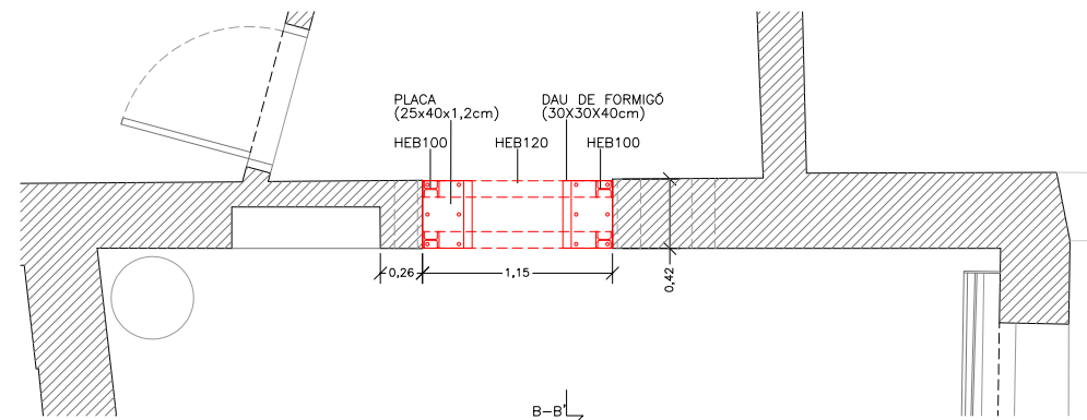
PLANTA PÒRTIC
