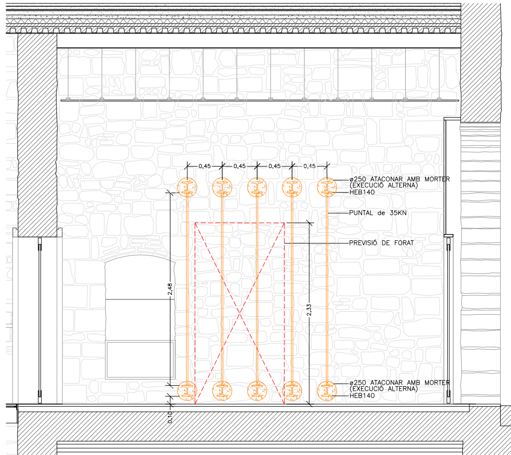
ALÇAT A-A' ESTINTOLAMENT PROVISIONAL
