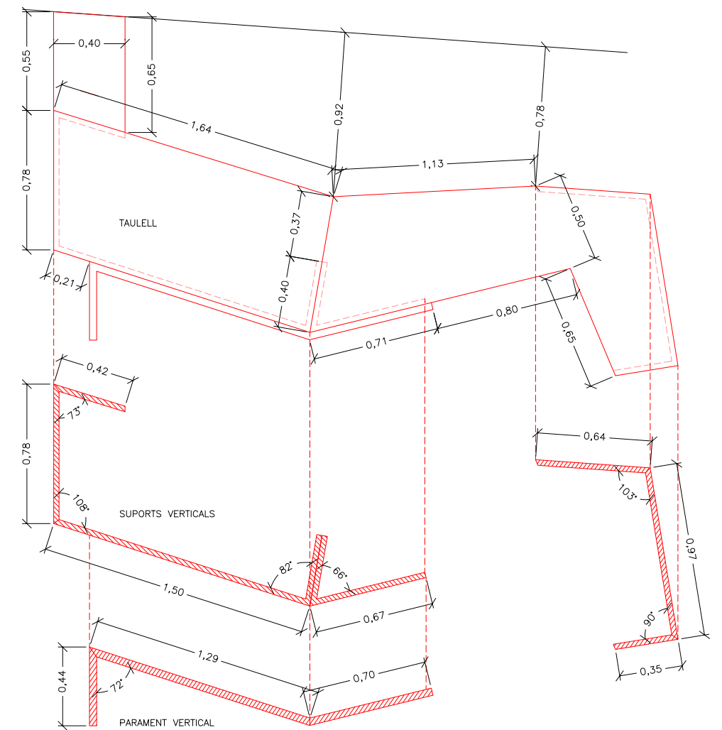
PLANTA ACOTADA PER PECES
