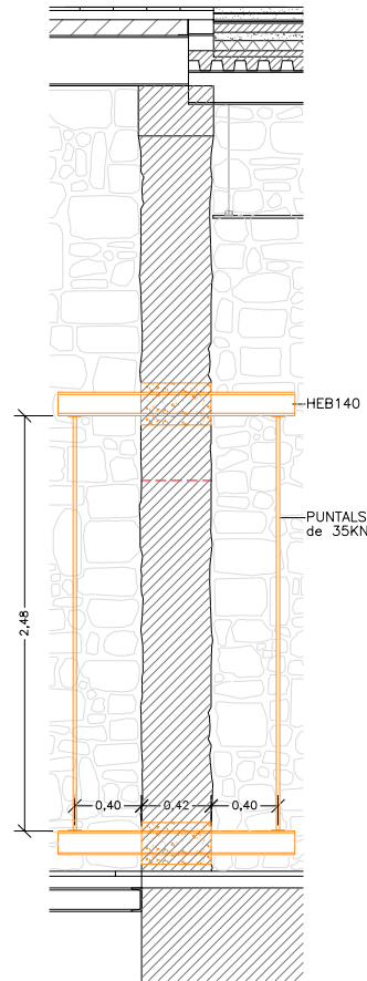
SECCIÓ B-B'
