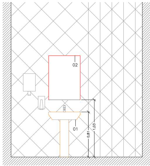
ALÇAT A-A' (ESTAT ACTUAL)
