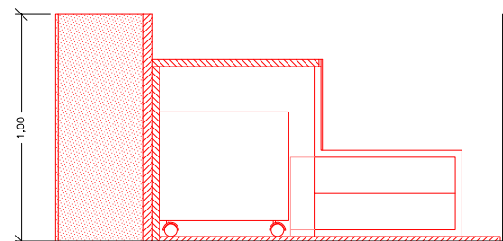
SECCIÓ B-B'
