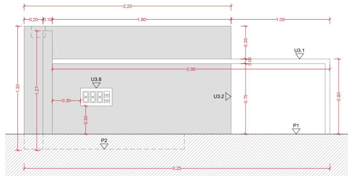
ALÇAT 03 DEL TAULELL MOSTRADOR
