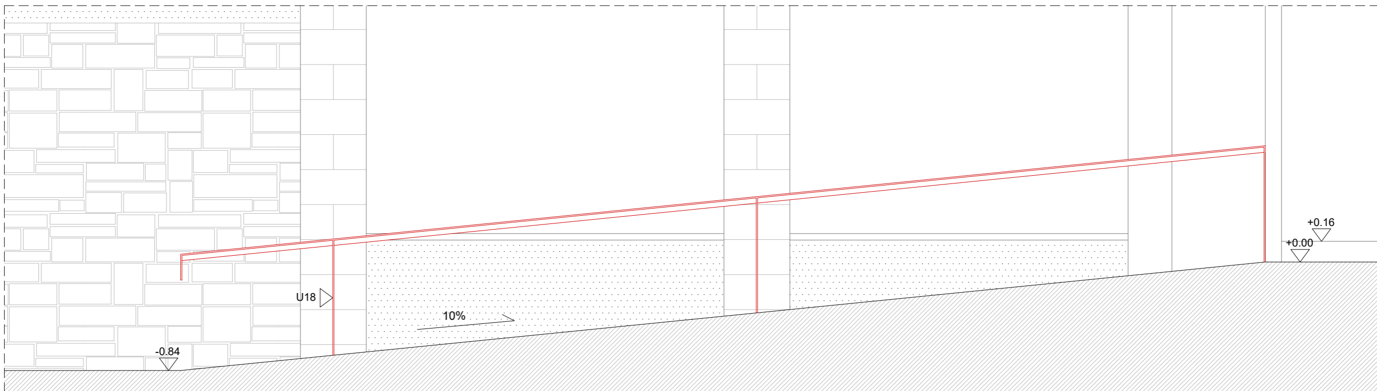
PROPOSTA PASSAMÀ RAMPA - SECCIÓ C-C'
