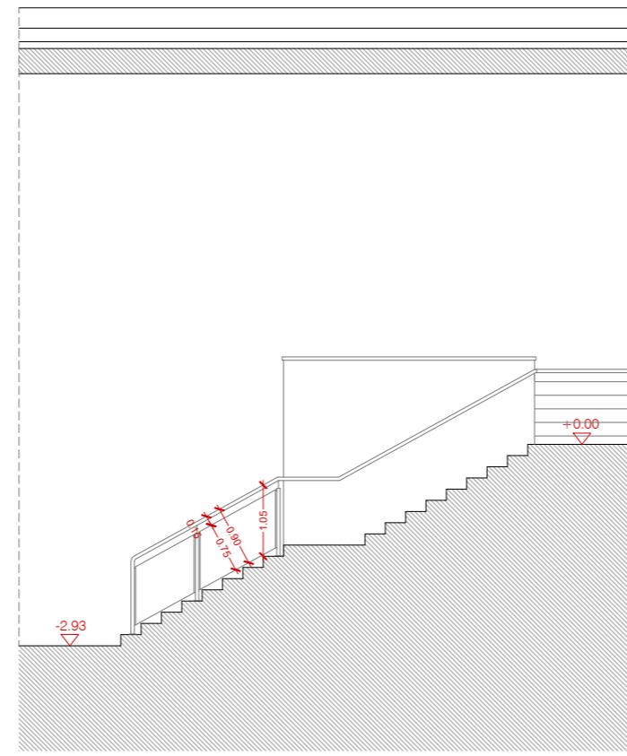
SECCIÓ B-B'
