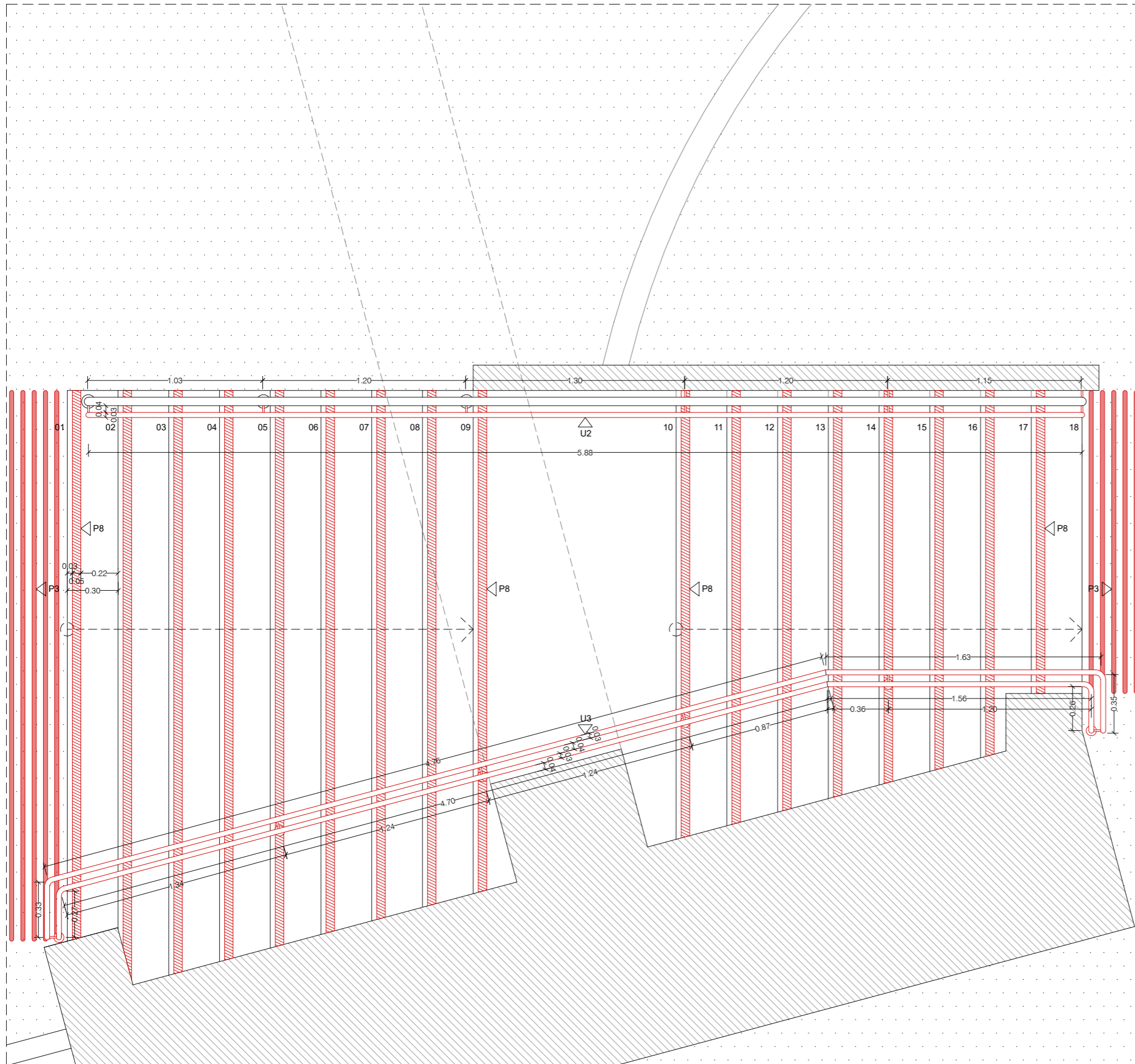
PROPOSTA ESCALA - PLANTA
