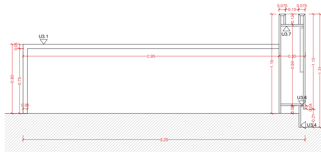
SECCIÓ LONGITUDINAL C-C'
