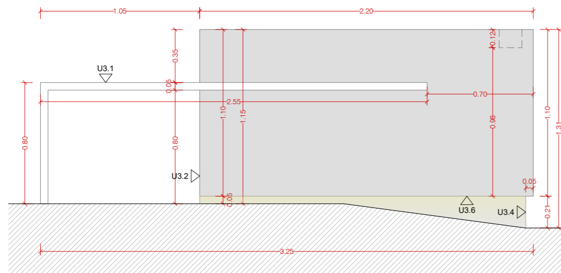
ALÇAT 01 DEL TAULELL MOSTRADOR
