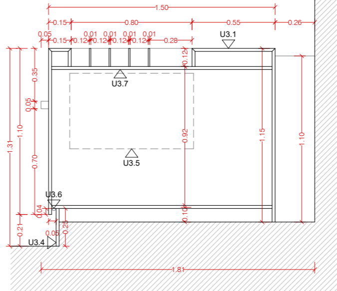
SECCIÓ TRANSVERSAL B-B'
