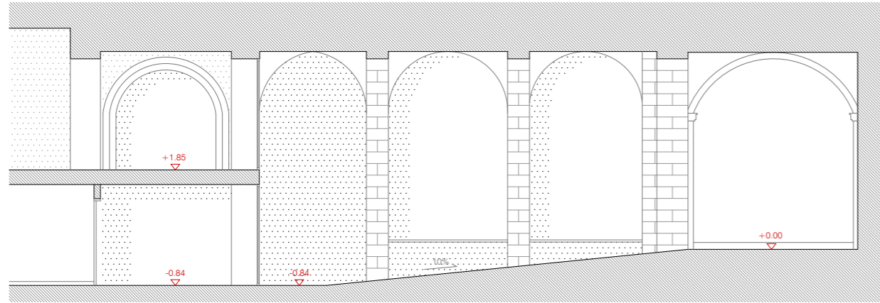
SECCIÓ TRANSVERSAL A-A'
