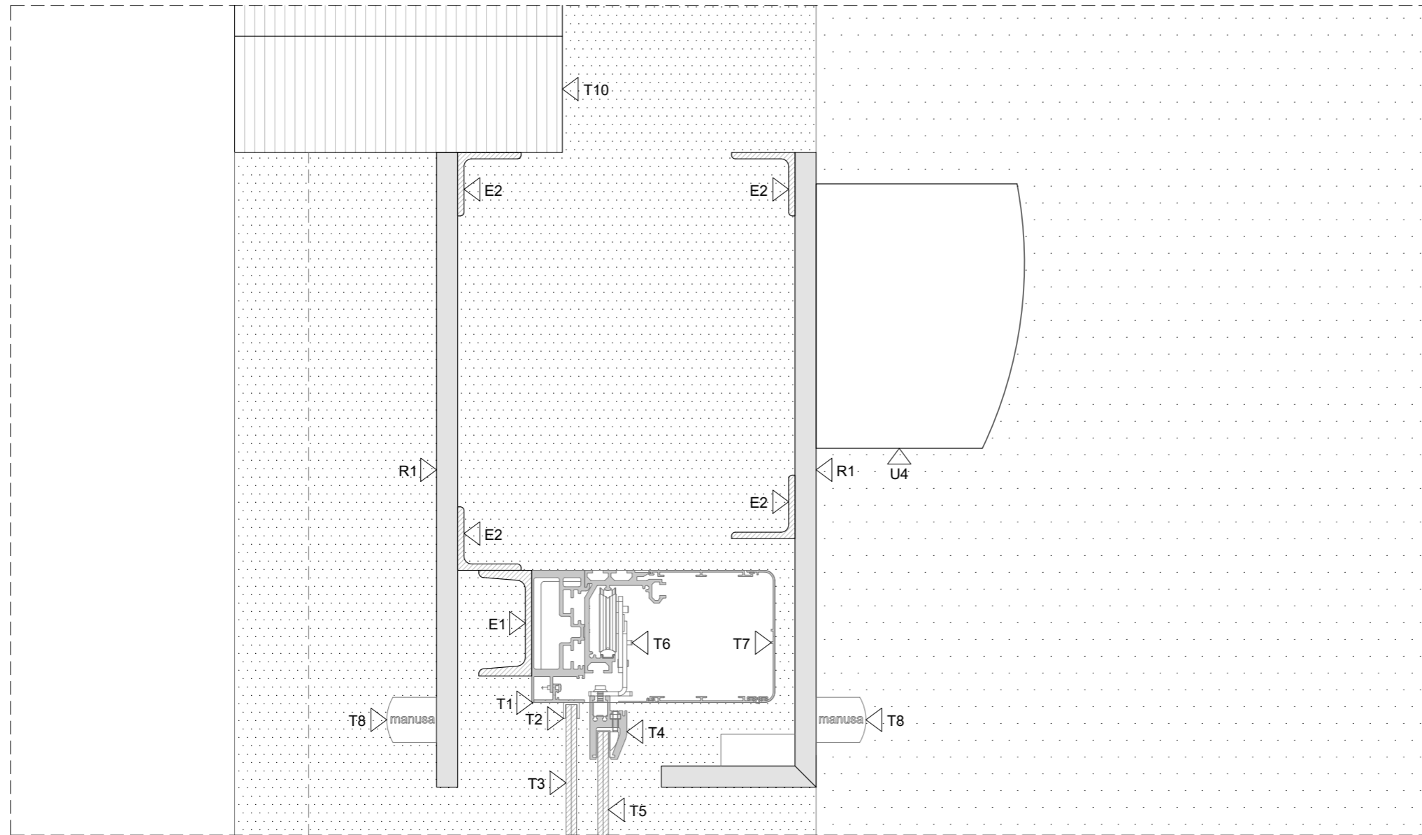
DETALL D01
