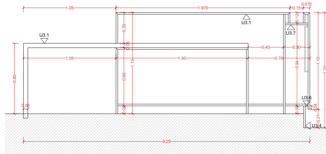
SECCIÓ LONGITUDINAL A-A'
