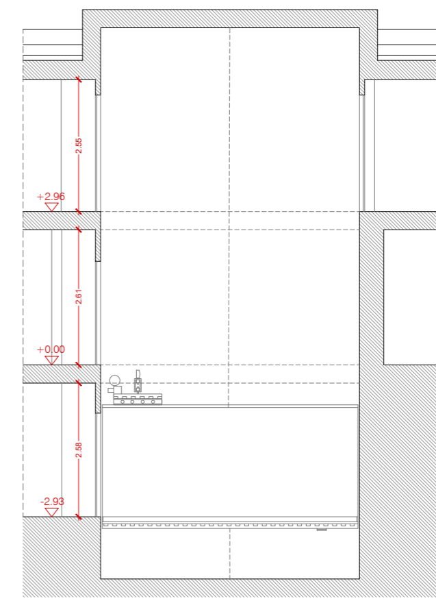
SECCIÓ C-C'
