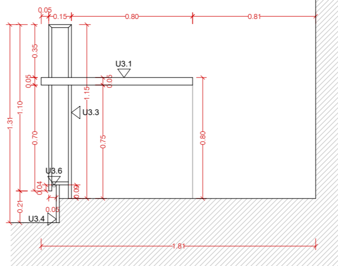
SECCIÓ TRANSVERSAL D-D'
