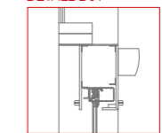
DETALL D01
