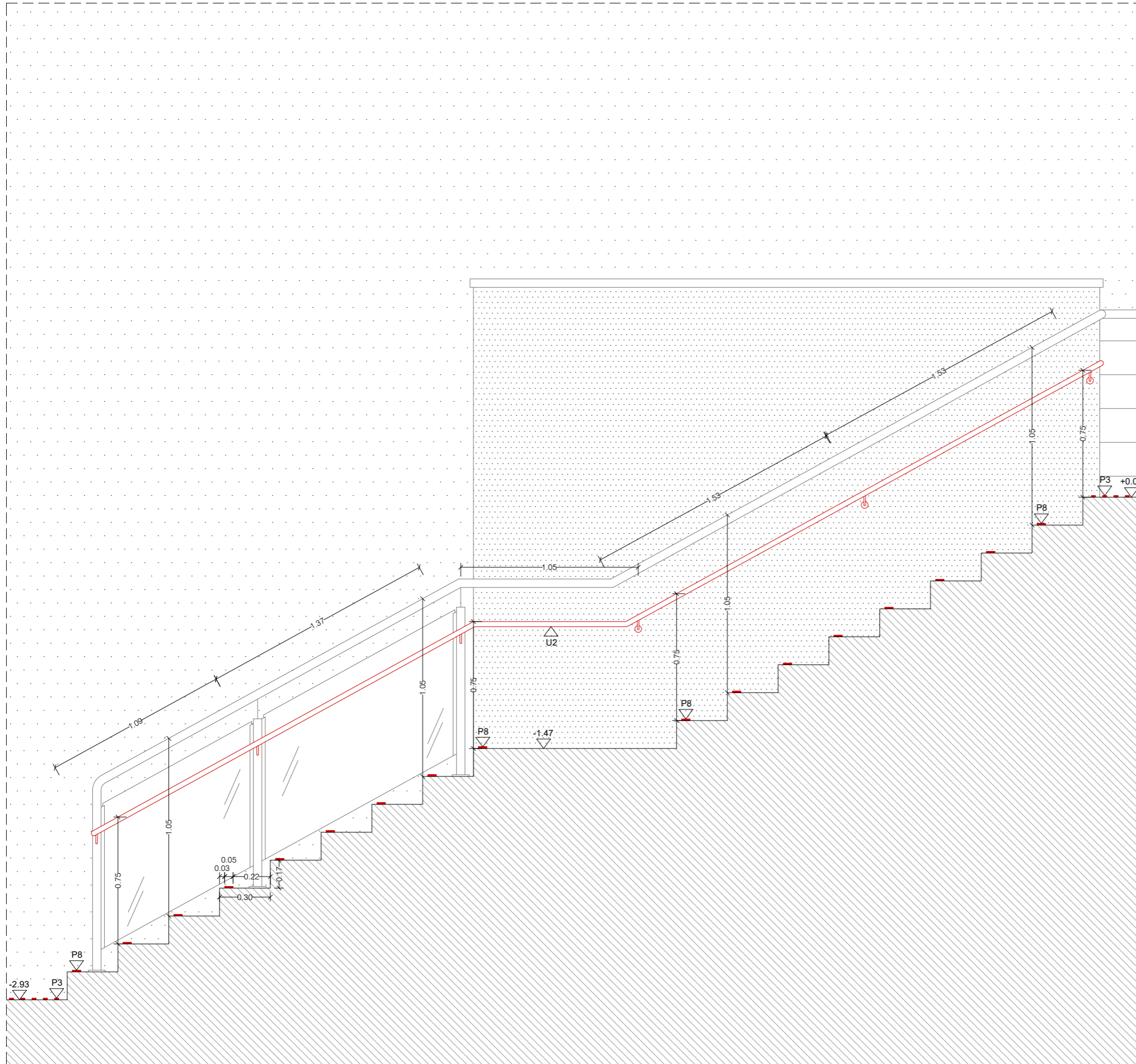
SECCIÓ A-A'
