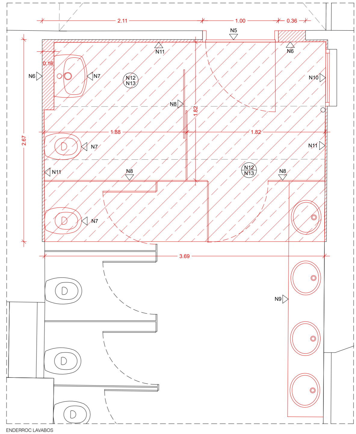
ENDERROC LAVABOS
