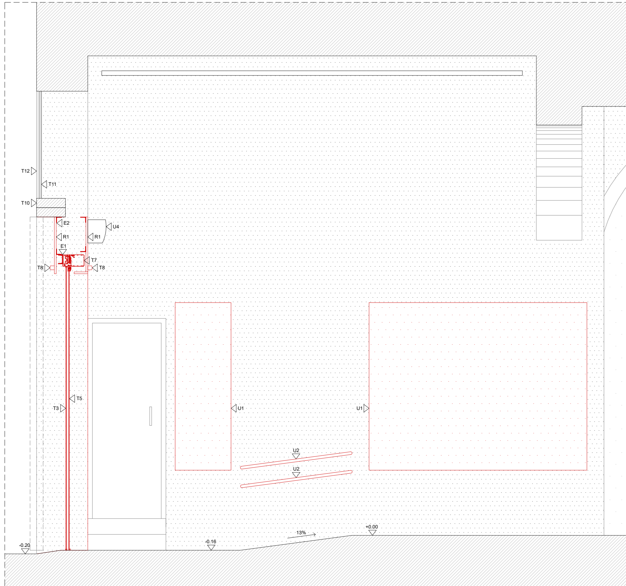
PROPOSTA VESTÍBUL - SECCIÓ A-A'
