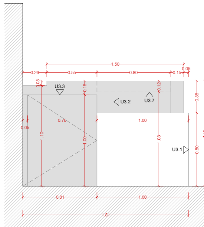
ALÇAT 04 DEL TAULELL MOSTRADOR
