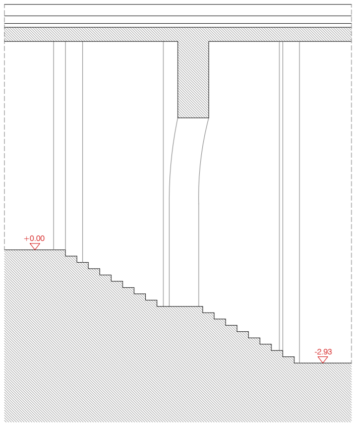
SECCIÓ A-A'
