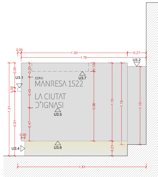
ALÇAT 02 DEL TAULELL MOSTRADOR
