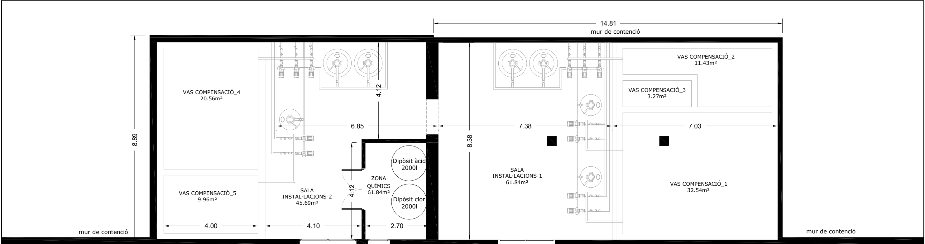
CARRER DE MIRALBÓ PLANTA BAIXA -PROPOSTA-
