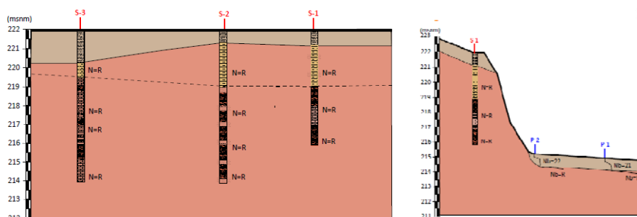
Figura 4 i Figura 5. Talls de correlació.
