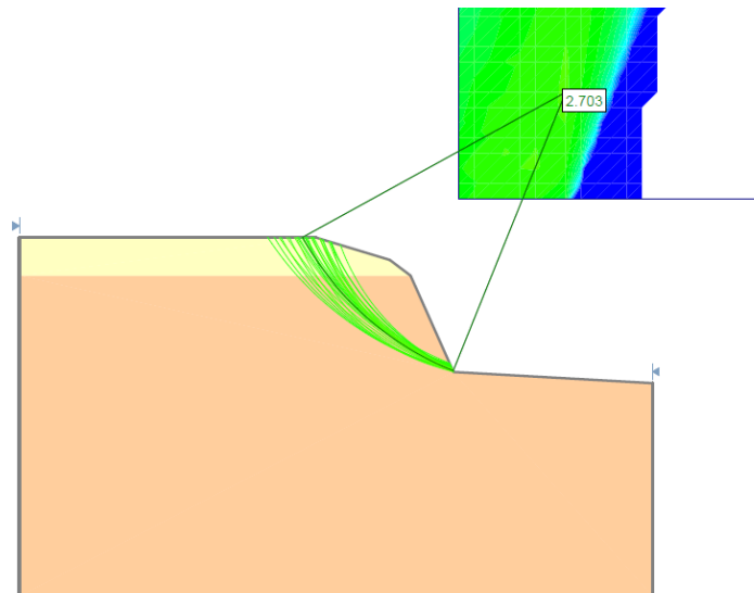
Figura 7. Detall de la sortida de l'SLIDE amb excavacions general del talús, amb pendents de 60°.
