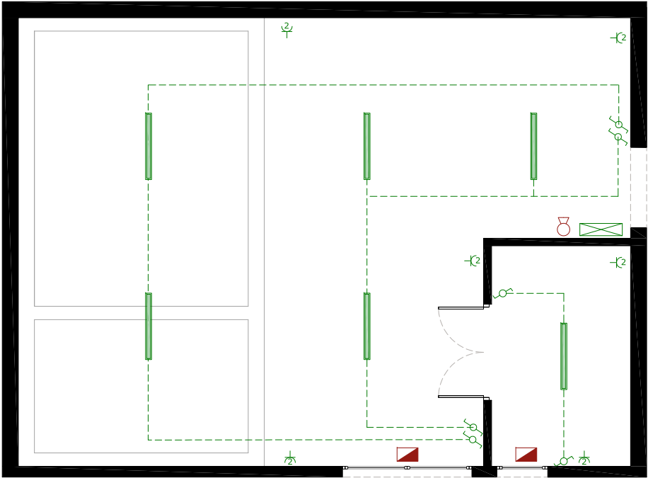
INSTAL·LACIÓ ELÈCTRICA -PROPOSTA-
