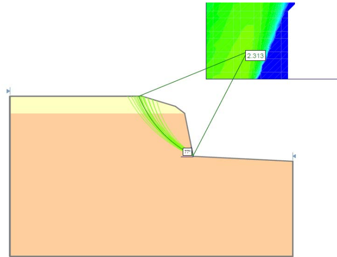
Figura 8. Detall de la sortida de l'SLIDE amb excavacions general del talús, amb pendents de 70°.
