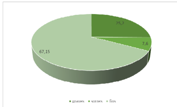
Gràfic 1. Distribució granulomètrica mitja dels trams més rics amb sorres i llims dels nivells de lutites.
