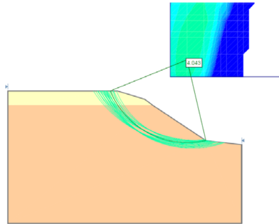
Figura 6. Detall de la sortida de l'SLIDE en la parcel·la actual.
