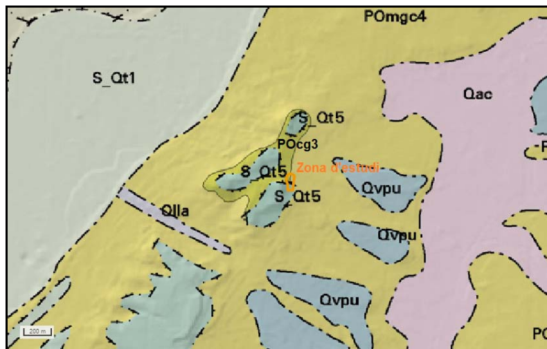
Figura 3. Mapa geològic a escala 1:50.000 de la zona en estudi (Font: ICGC).
