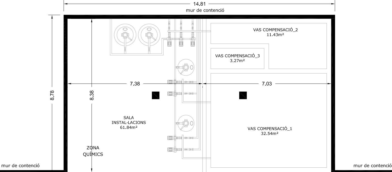
CARRER DE MIRALBÓ PLANTA BAIXA -ESTAT ACTUAL-
