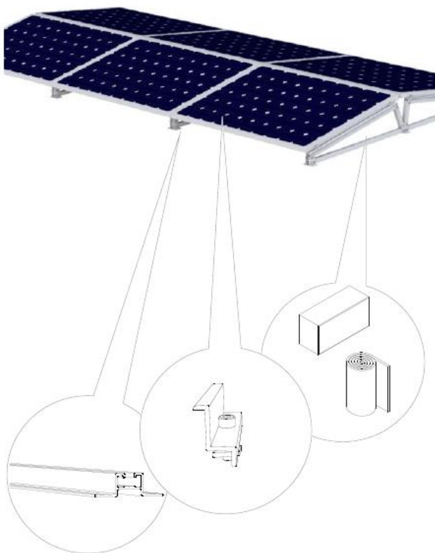
Il·lustració 5. Tipus d'estructura utilitzada
