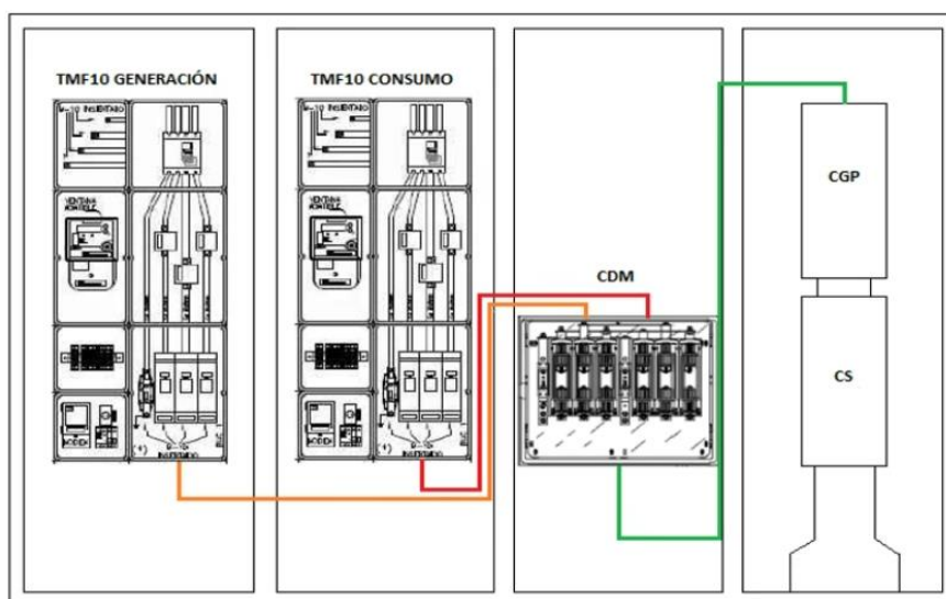
II-lustració 9. Esquema de muntatge
