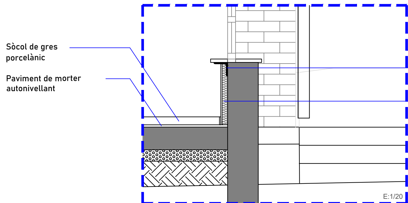
SECCIÓ A-A'
