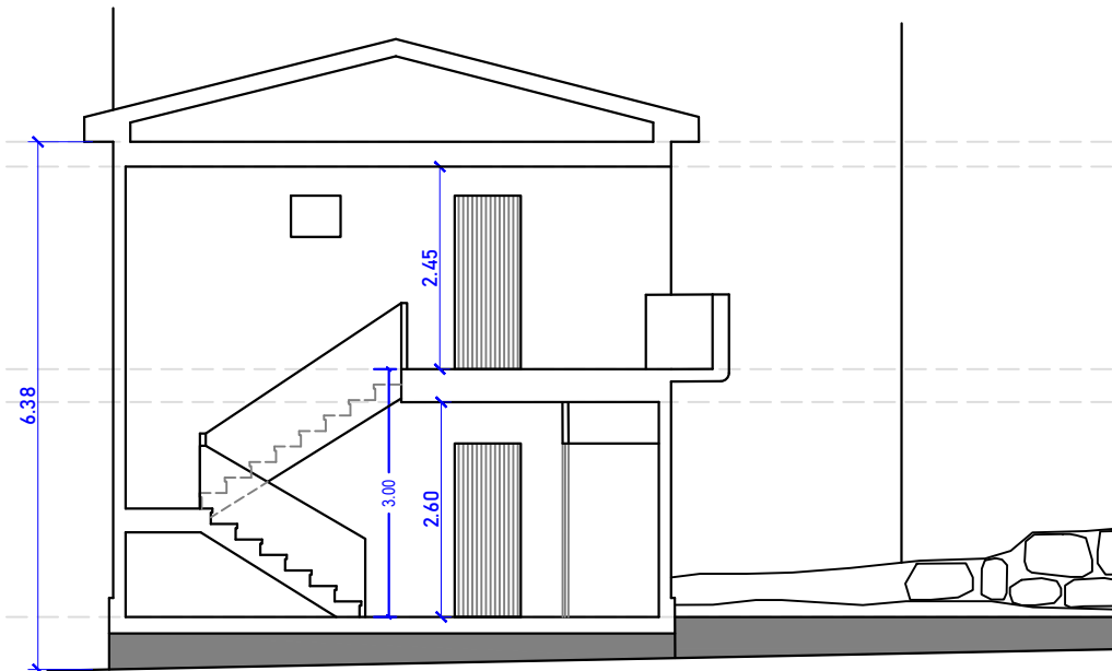
SECCIÓ A-A'
