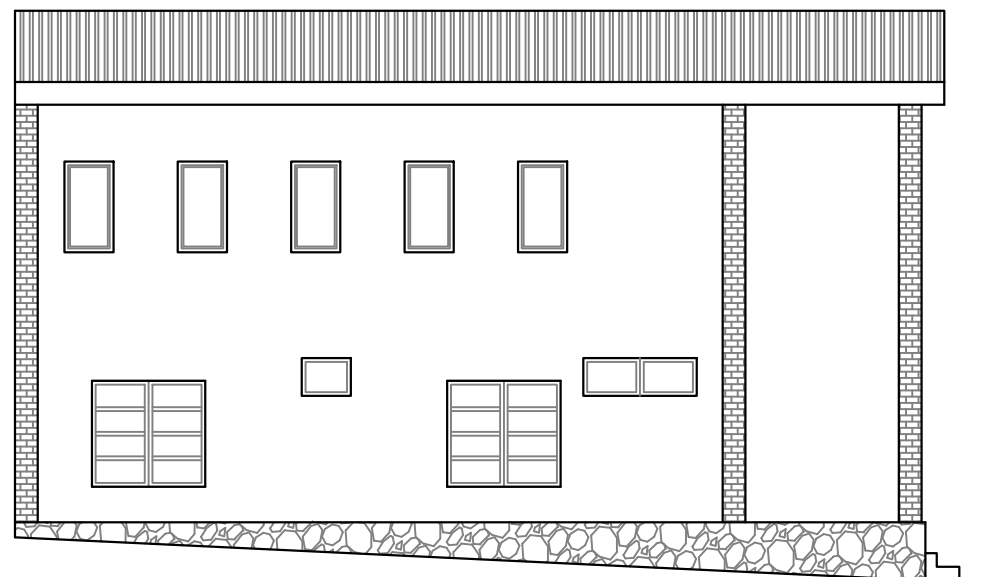
ALÇAT NORD
