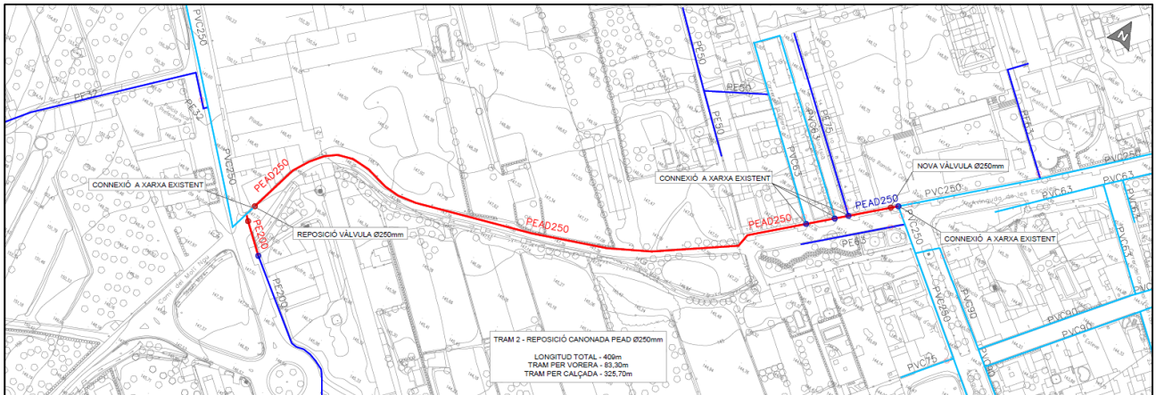
Figura 3. Xarxa d'abastament projectada per al tram 2.
