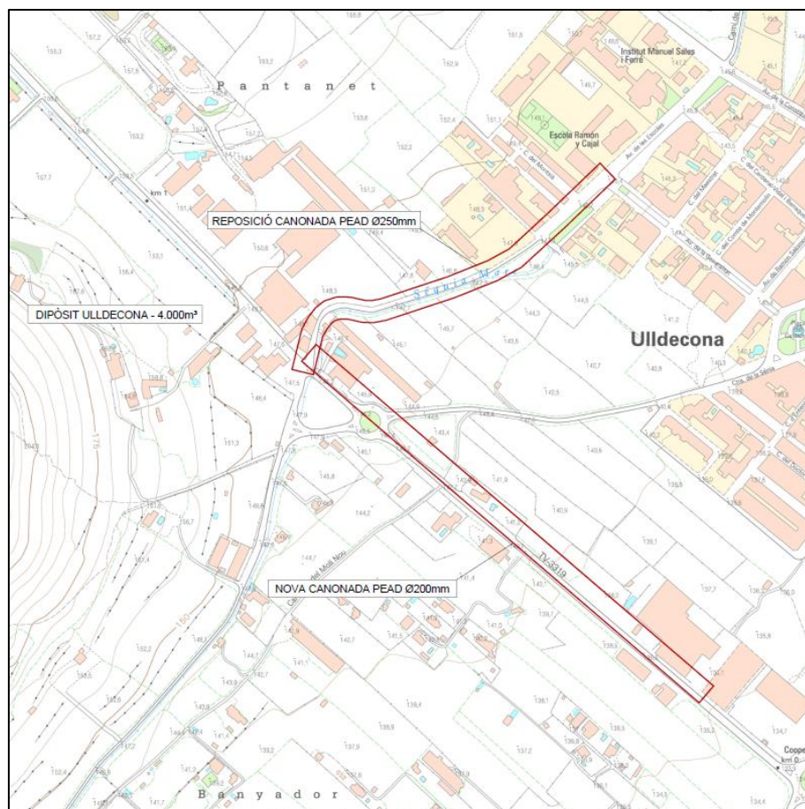
Figura 1. Emplaçament dels dos trams d'instal·lació de canonada d'aigua potable.
