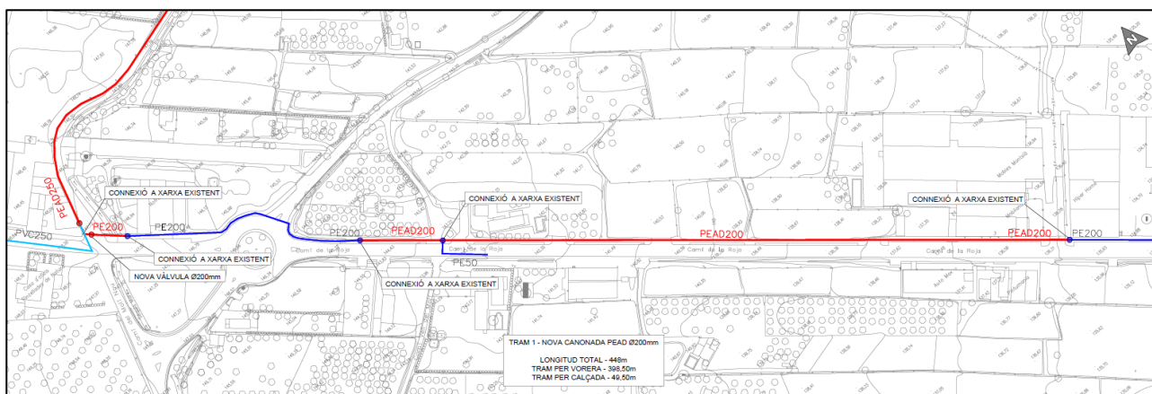
Figura 2. Xarxa d'abastament projectada per al tram 1.
