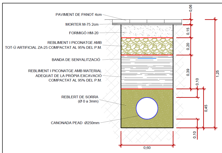
Figura 6. Secció tipus de la rasa en vorera per a la canonada de PEAD (polietilè d'alta densitat) de diàmetre nominal 250 mm.
