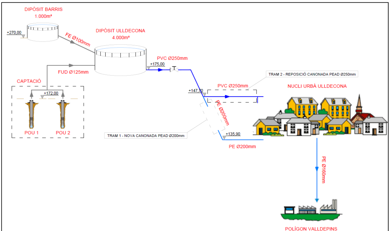
Figura 4. Esquema vertical de la instal·lació.
