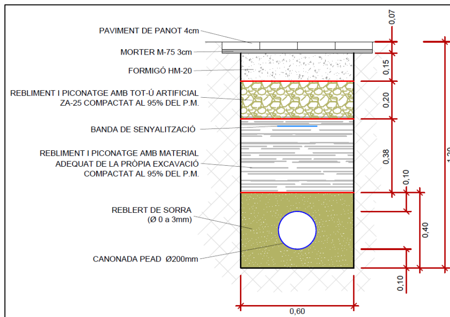
Figura 8. Secció tipus de la rasa en vorera per a la canonada de PEAD (polietilè d'alta densitat) de diàmetre nominal 200 mm.
