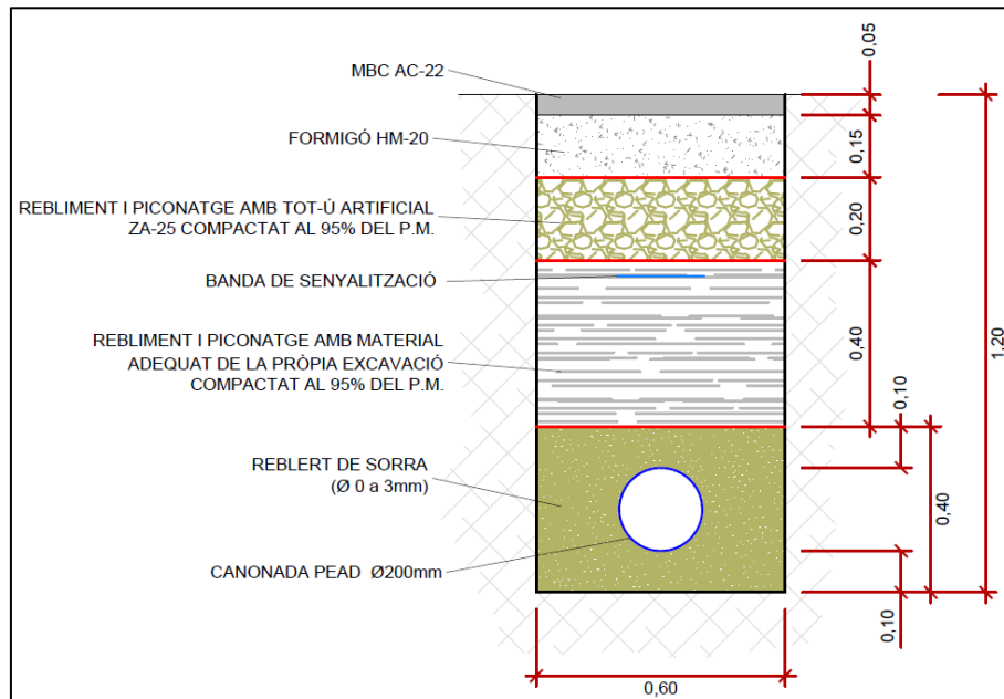
Figura 7. Secció tipus de la rasa en calçada per a la canonada de PEAD (polietilè d'alta densitat) de diàmetre nominal 200 mm.
