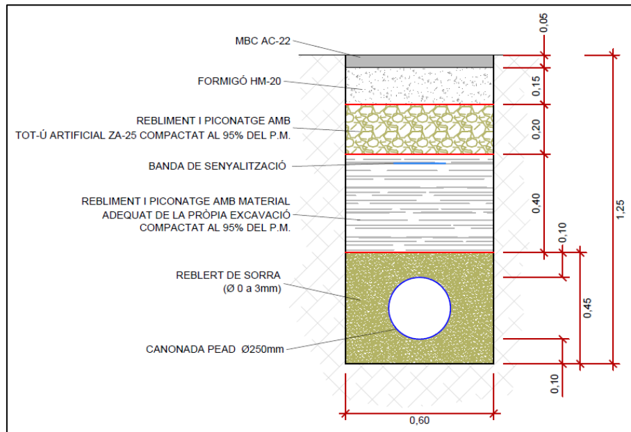
Figura 5. Secció tipus de la rasa en calçada per a la canonada de PEAD (polietilè d'alta densitat) de diàmetre nominal 250 mm.
