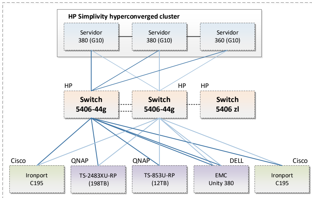
Figura 2 – Arquitectura actual sistemes d'informació Ajuntament
