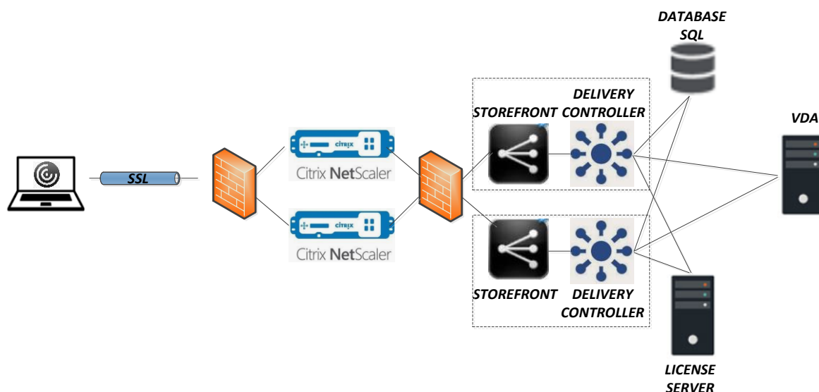
Figura 3 – Arquitectura sistema de virtualització d'escriptoris Citrix
