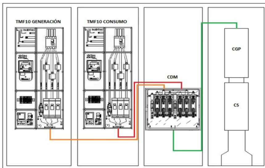
Il·lustració 9. Esquema de muntatge
