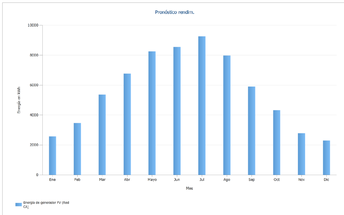
II-lustració 8. Generació fotovoltaica anual
