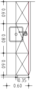
MFA 3. Office format per mobles alts i baixos segons dibuix, inclòs pica, moble baix amb 4 calaixos i moble alt preparat per a microneos.
