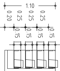
P9 3 moduls de 100 cm amb plafons d'acabat als extrems i superior P10 2 moduls de 90 cm amb plafons d'acabat als extrems P11 4 moduls de 90 cm amb plafons d'acabat als extrems P12 3 mòduls de 80 i 2 mòduls de 100 amb plafons d'acabat als extrems i superior P13 2 mòduls de 80 i 3 mòduls de 100 amb plafons d'acabat als extrems i superior P14 3 mòduls de 100 amb plafons d'acabat als extrems i superior
