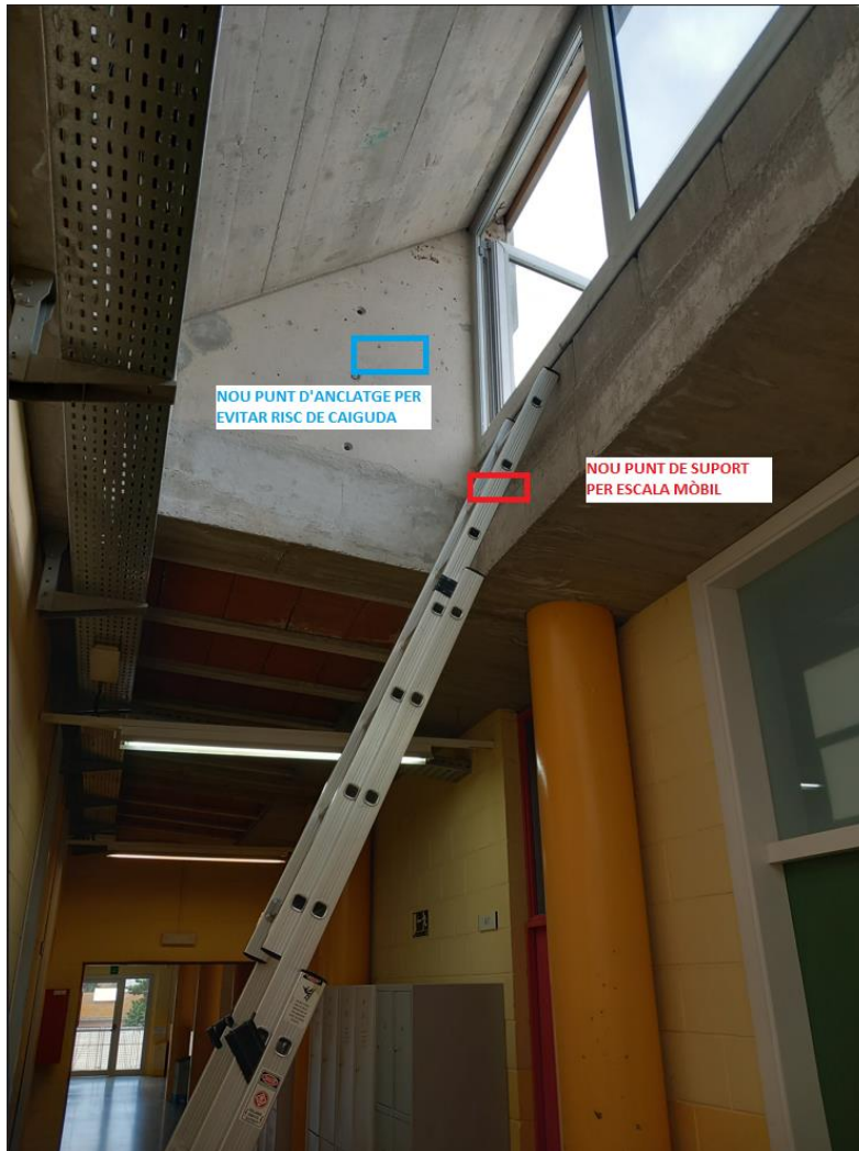
Il·lustració 16. Proteccions col·lectives i accessos durant la fase d'execució
