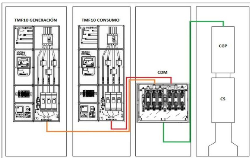
Il·lustració 10. Esquema de muntatge
