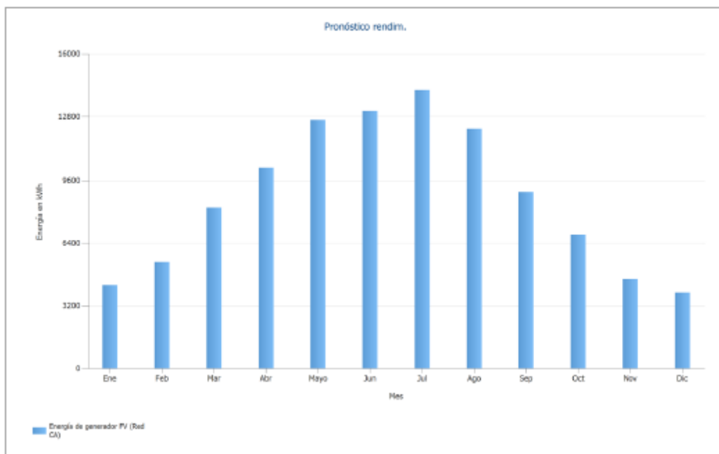
Il·lustració 8. Generació fotovoltaica anual
