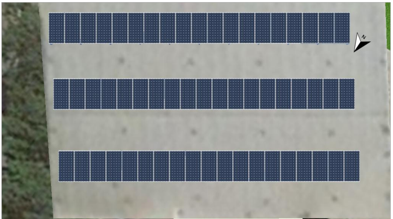
Figura: 2. Superficie fotovoltaica - Edificio a discreción 04-Superficie a ocupar Noroeste
