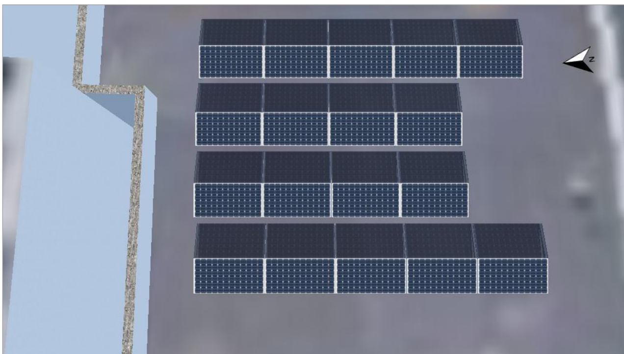
Figura: 2. Superficie fotovoltaica - Edificio a discreción 06-Superficie fotovoltaica Oeste
