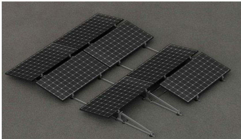
Figura 4 Estructura orientada E-O amb inclinació 10° i subjecte en costat llarg. Font: Sunfer
