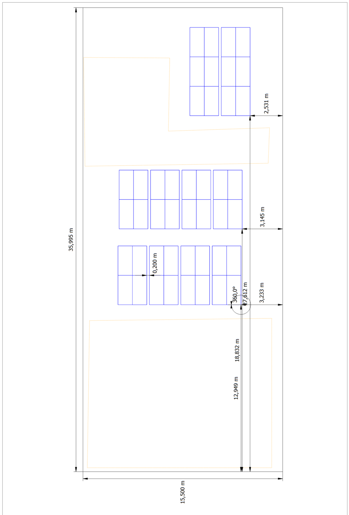
Figura: Coberta Gimnàs - Superfície del tejado sudeste
