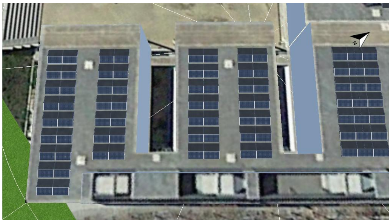
Figura: 2. Superficie fotovoltaica - Coberta Aulari-Superficie fotovoltaica sudeste
